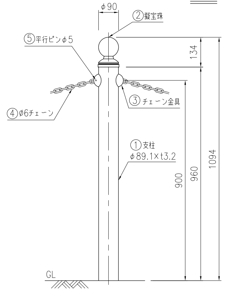
支柱図
