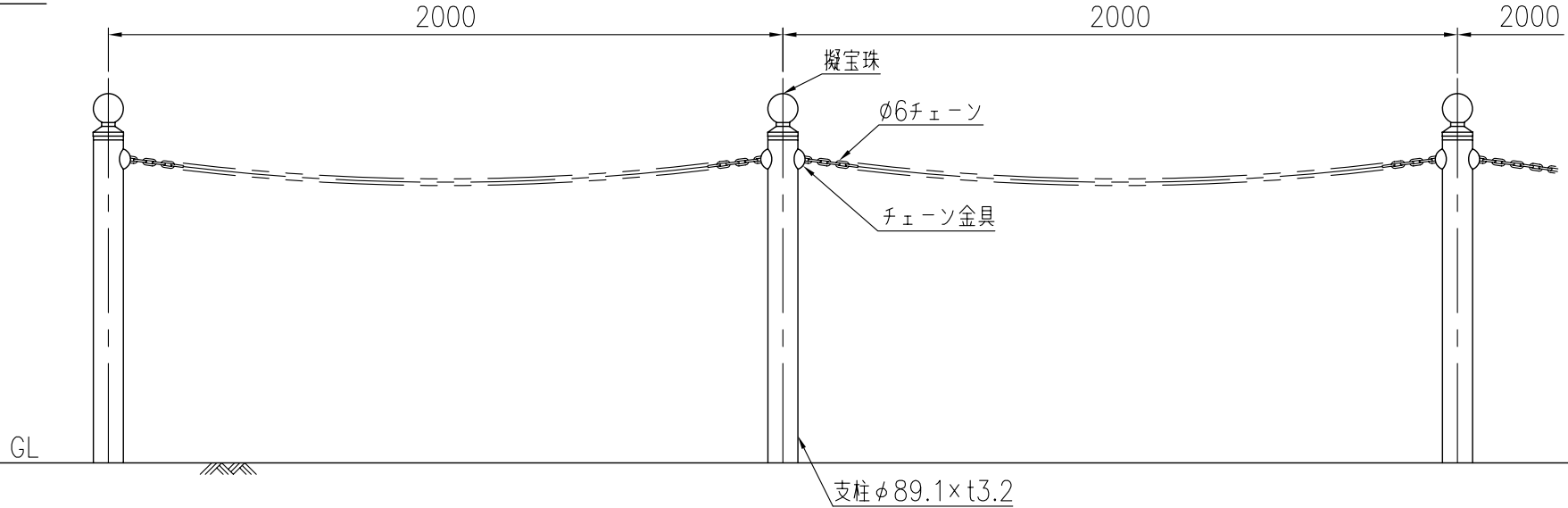
設置図
