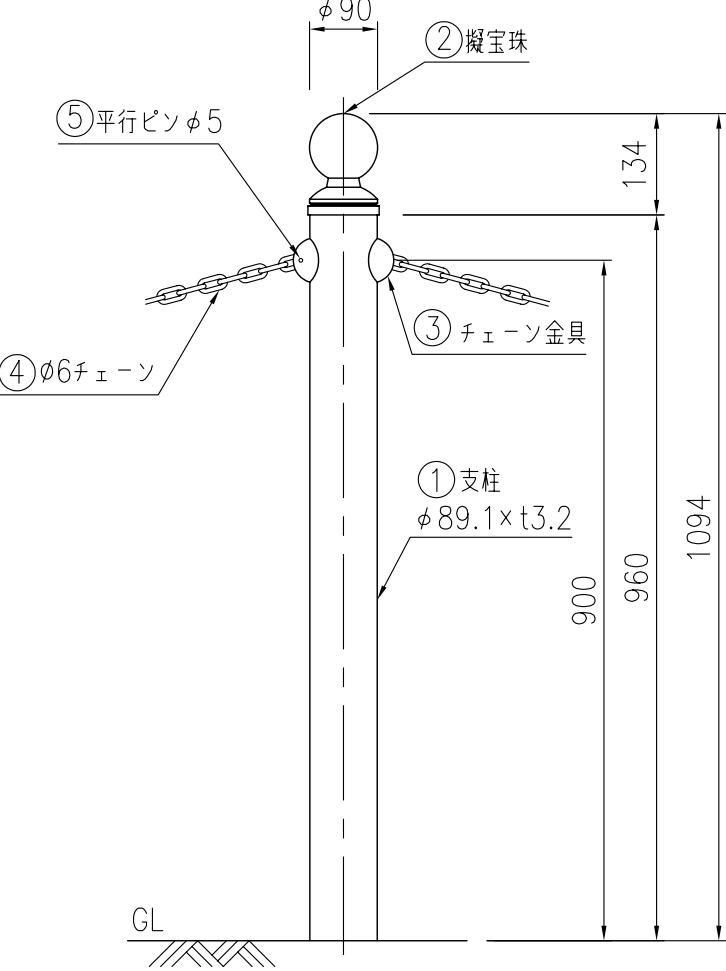
支柱図
