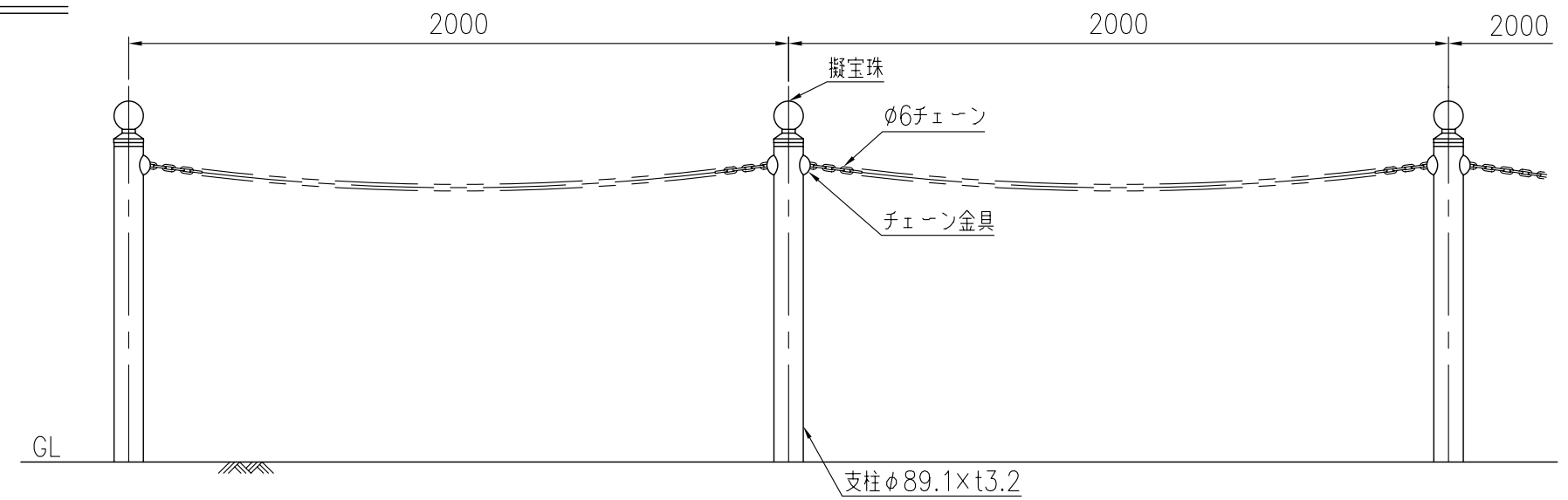
設置図
