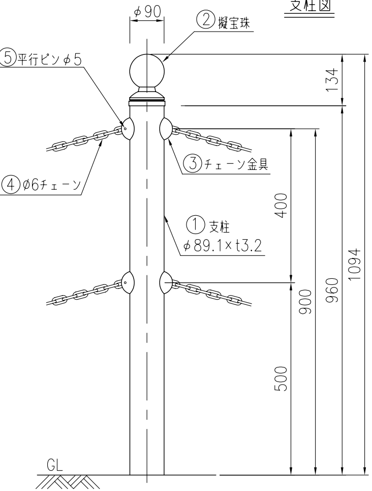
支柱図
