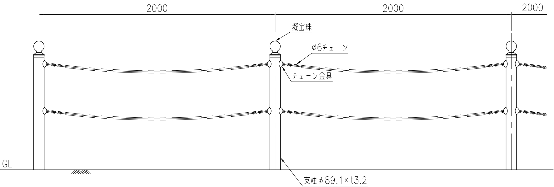
設置図
