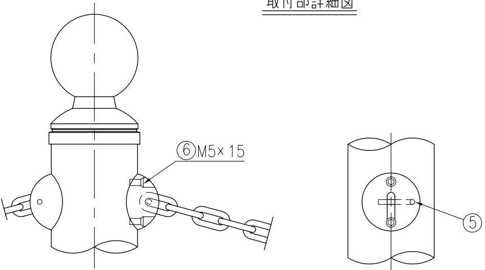
取付部詳細図
