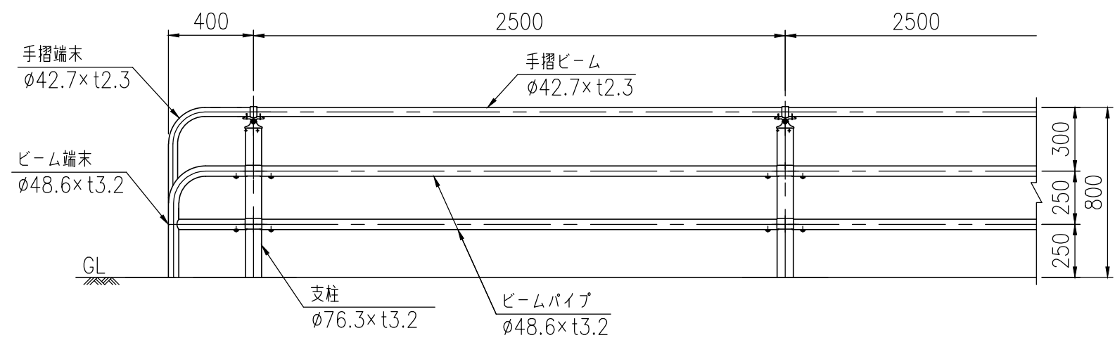
設置図 (1/25)
