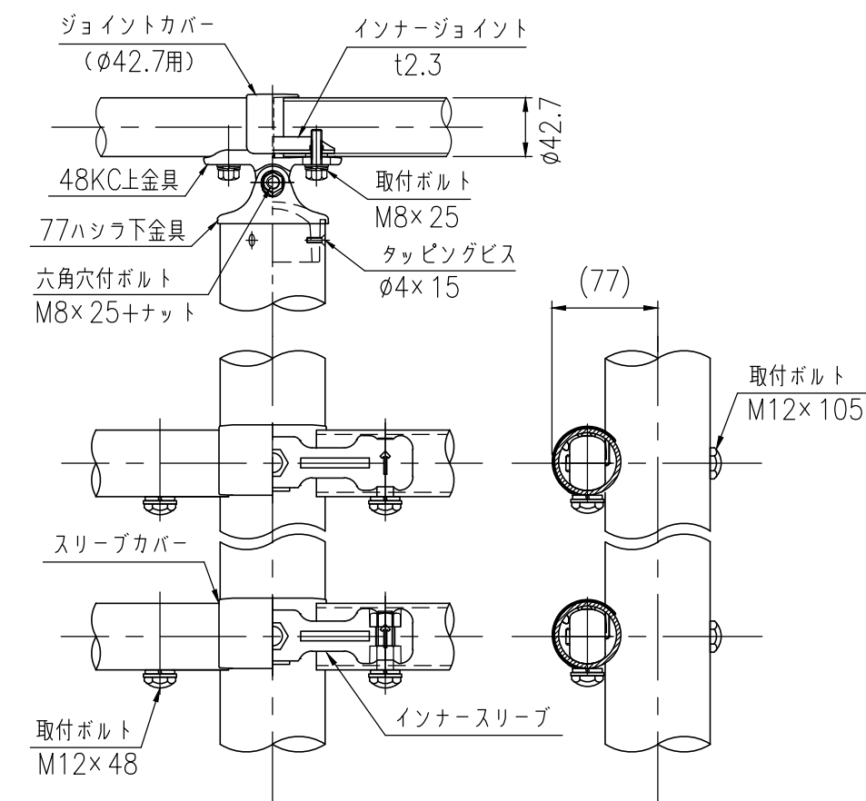
ビームパイプ詳細図 (1/10)
