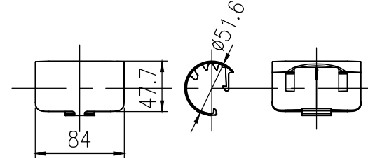
スリーブカバー詳細図 (1/5)
