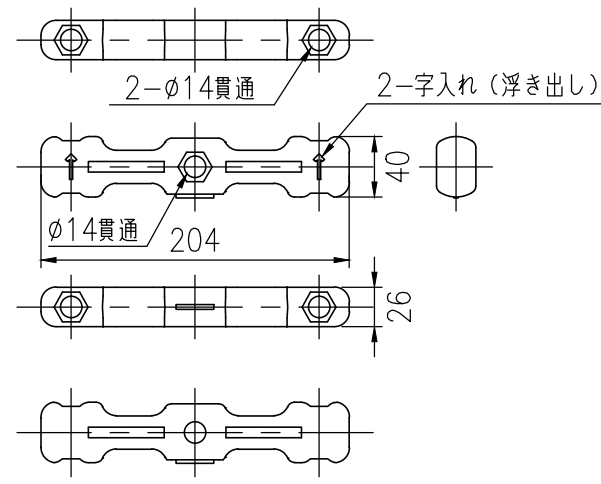
インナースリーブ詳細図 (1/5)
