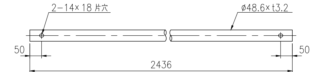
ビームパイプ詳細図 (1/10)
