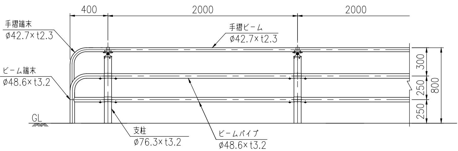
設置図 (1/25)
