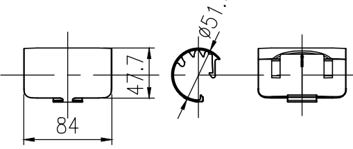
スリーブカバー詳細図 (1/5)
