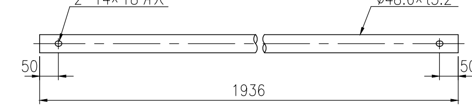
ビームパイプ詳細図 (1/10)
