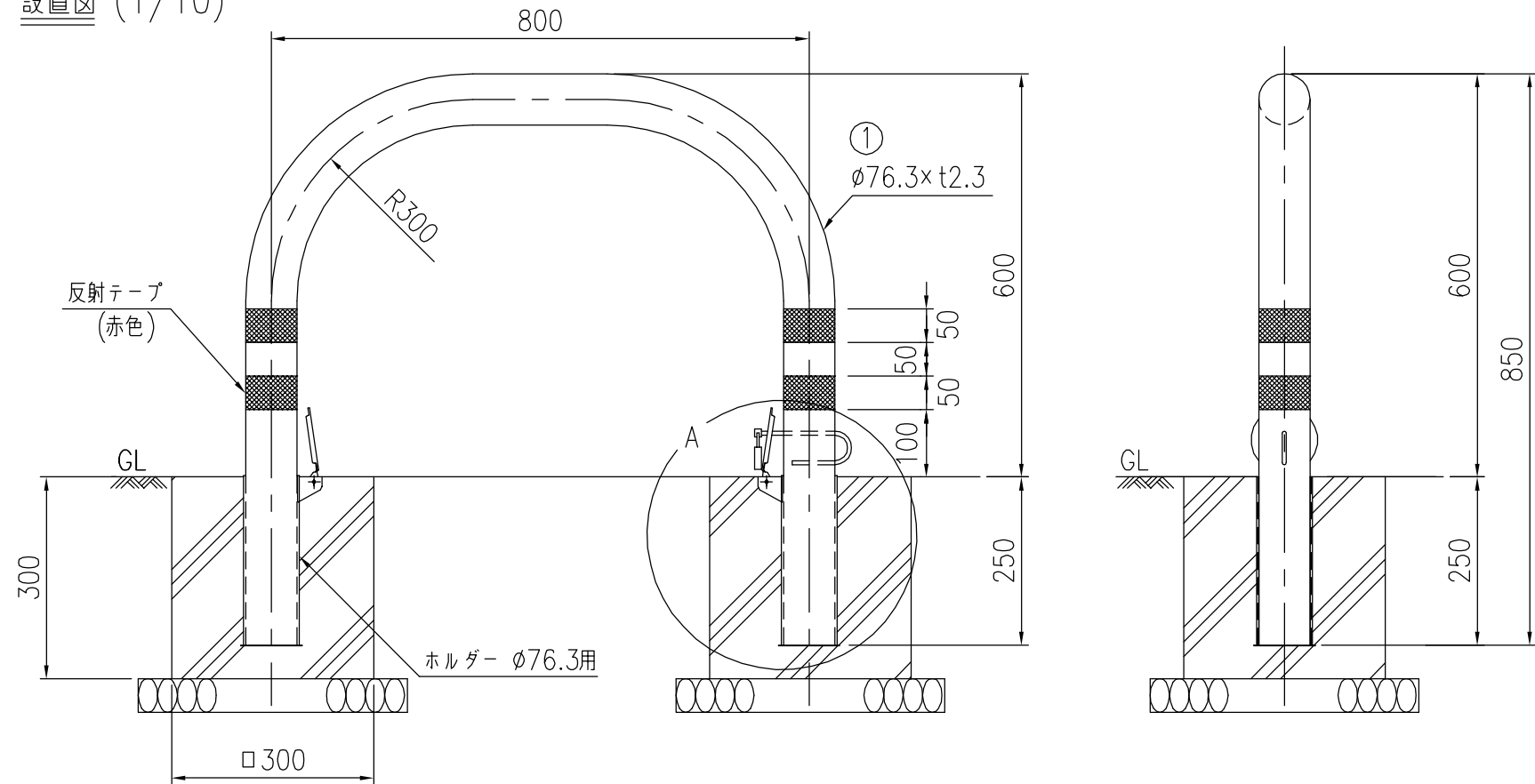
設置図 (1/10)
