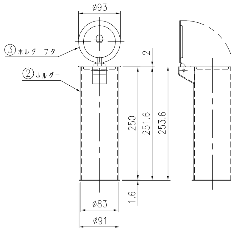
ホルダー詳細図 (1/5)
