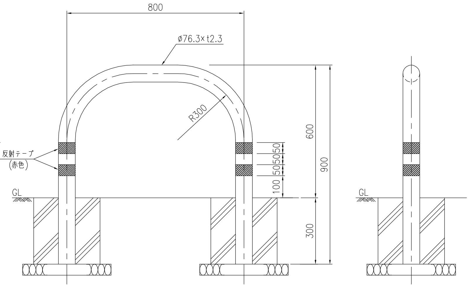
設置図 (1/10)
