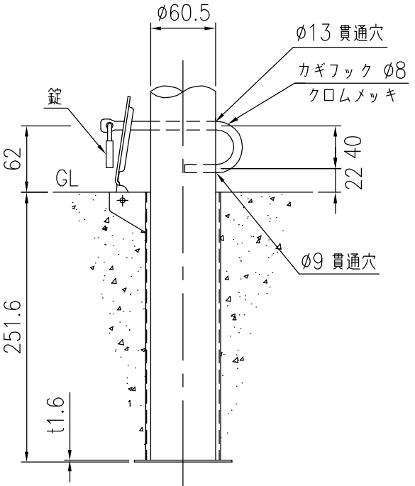
A 部詳細図 (1/5)
