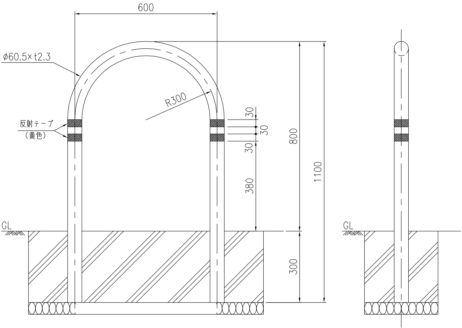
設置図 (1/10)
