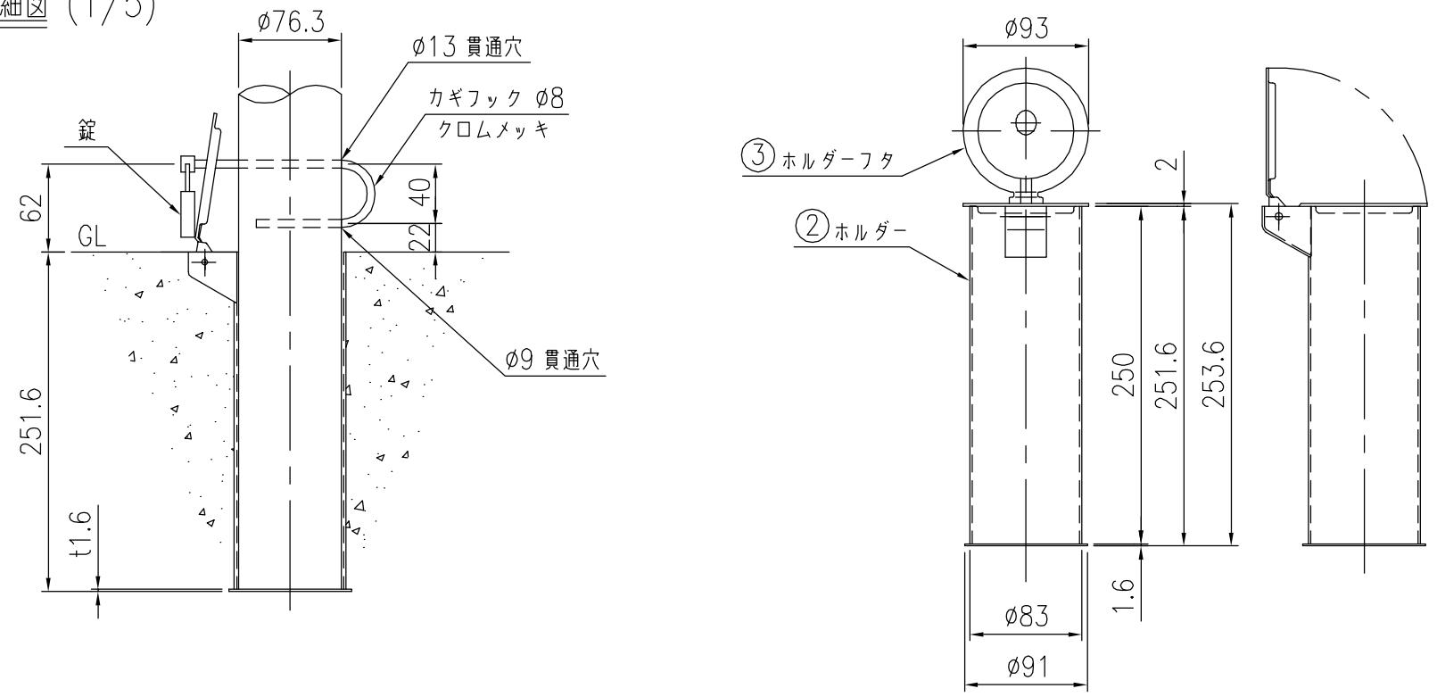
ホルダー詳細図 (1/5)
