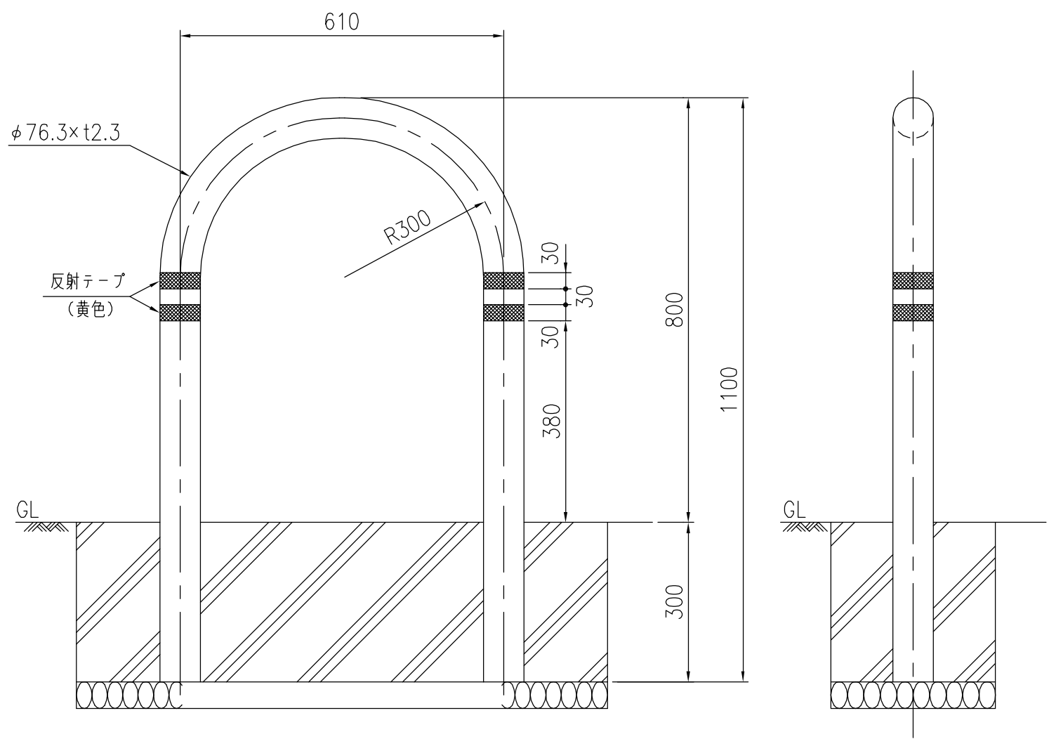
設置図 (1/10)
