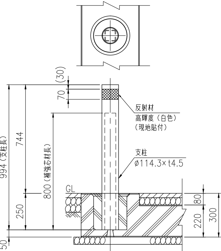
支柱設置図(1/15)
