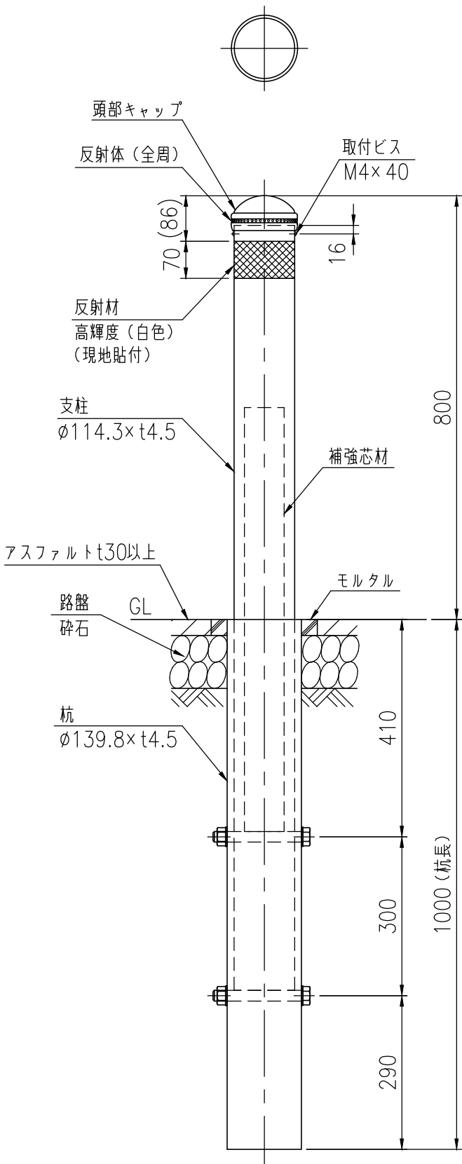
BSK-F114E(1/10)
