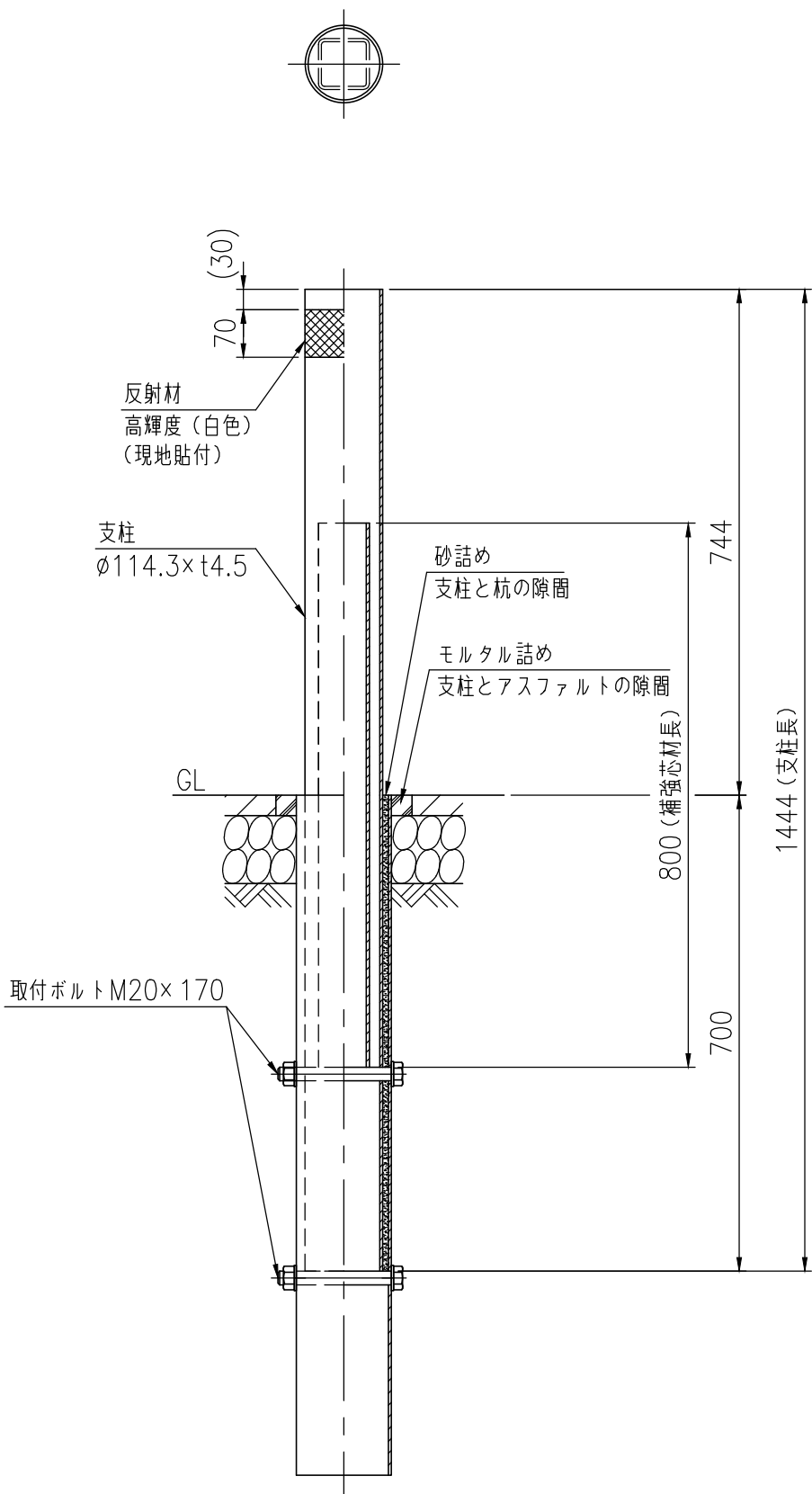
支柱設置図(1/10)
