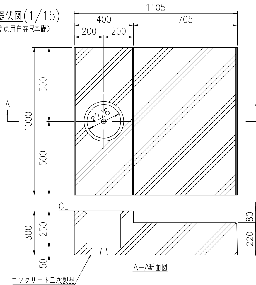
支柱設置図(1/15)
