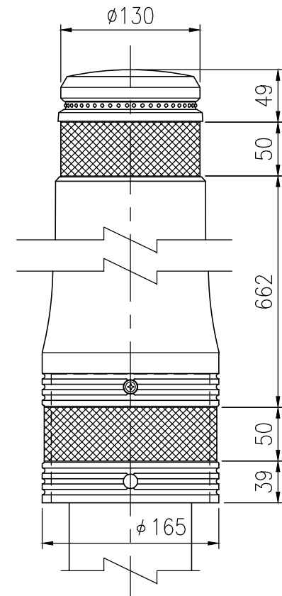
反射シート貼付部詳細図(1/5)
