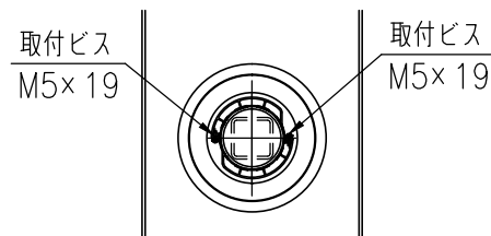
支柱設置図(1/15)
