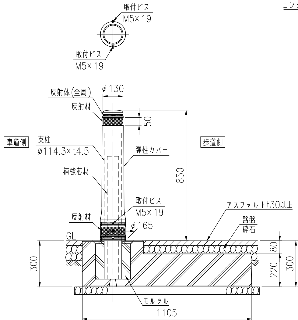
BSK-11TK(1/15)
