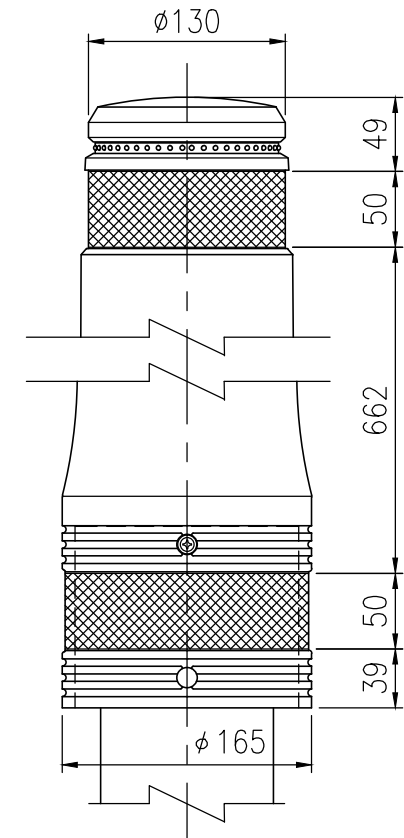
反射シート貼付部詳細図(1/5)
