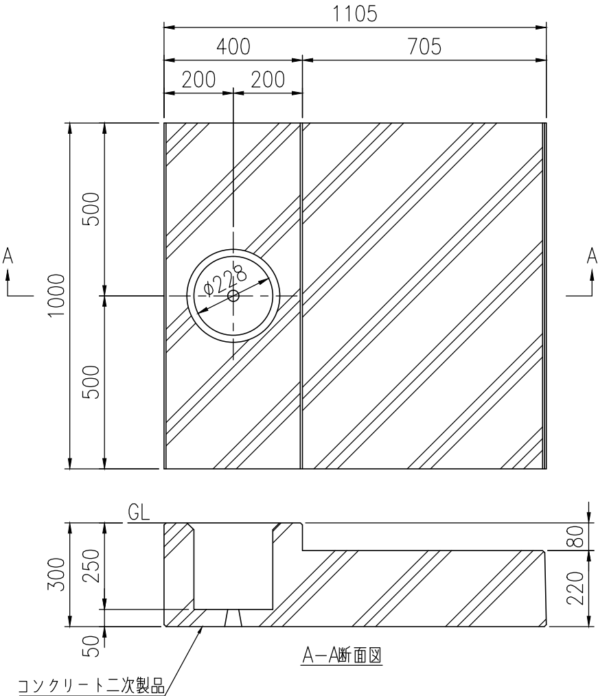
基礎伏図(1/15) (交差点用自在R基礎)
