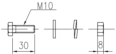
取付ボルト (1/3)
