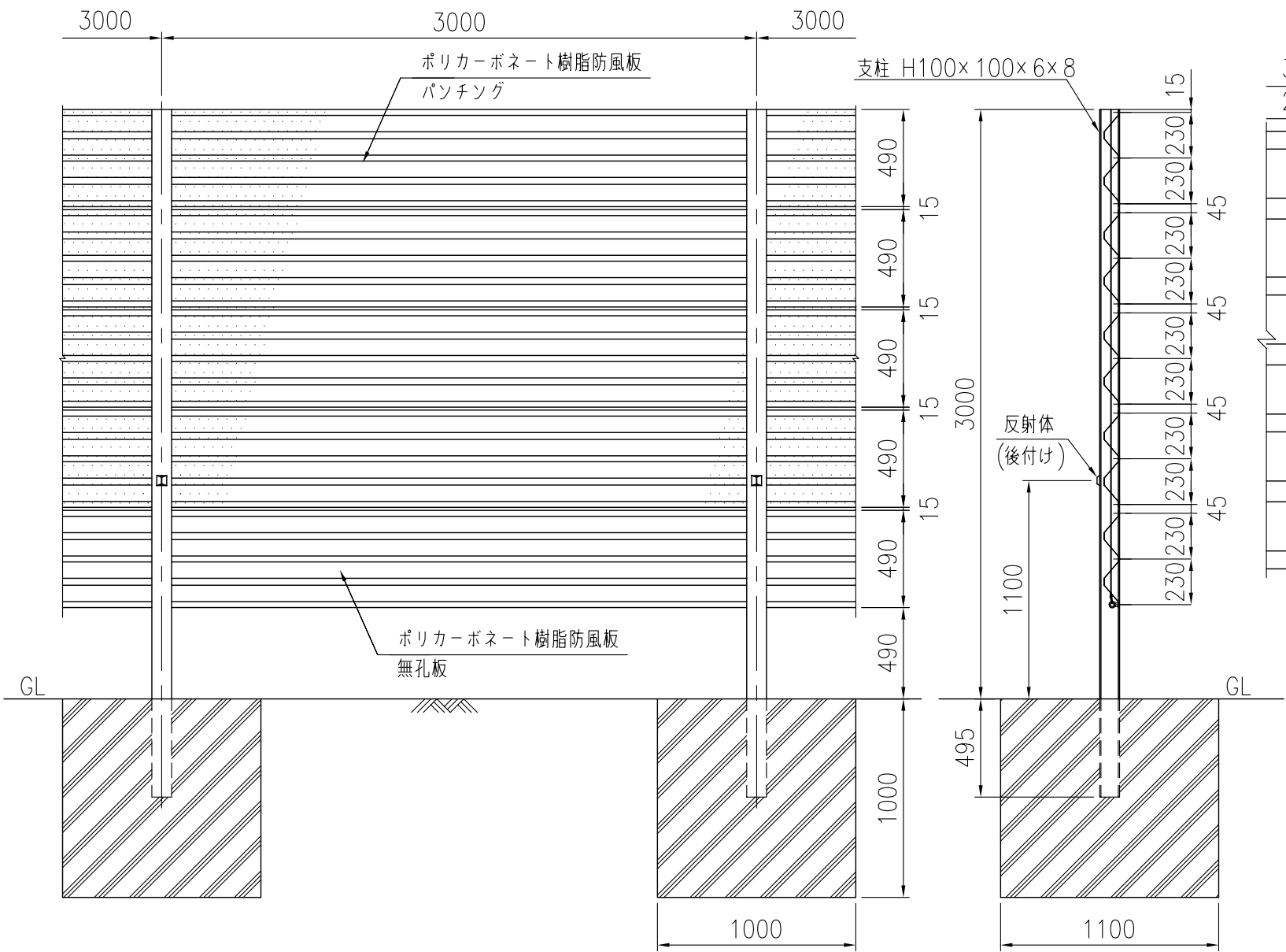
パンチングレール (1/15)
