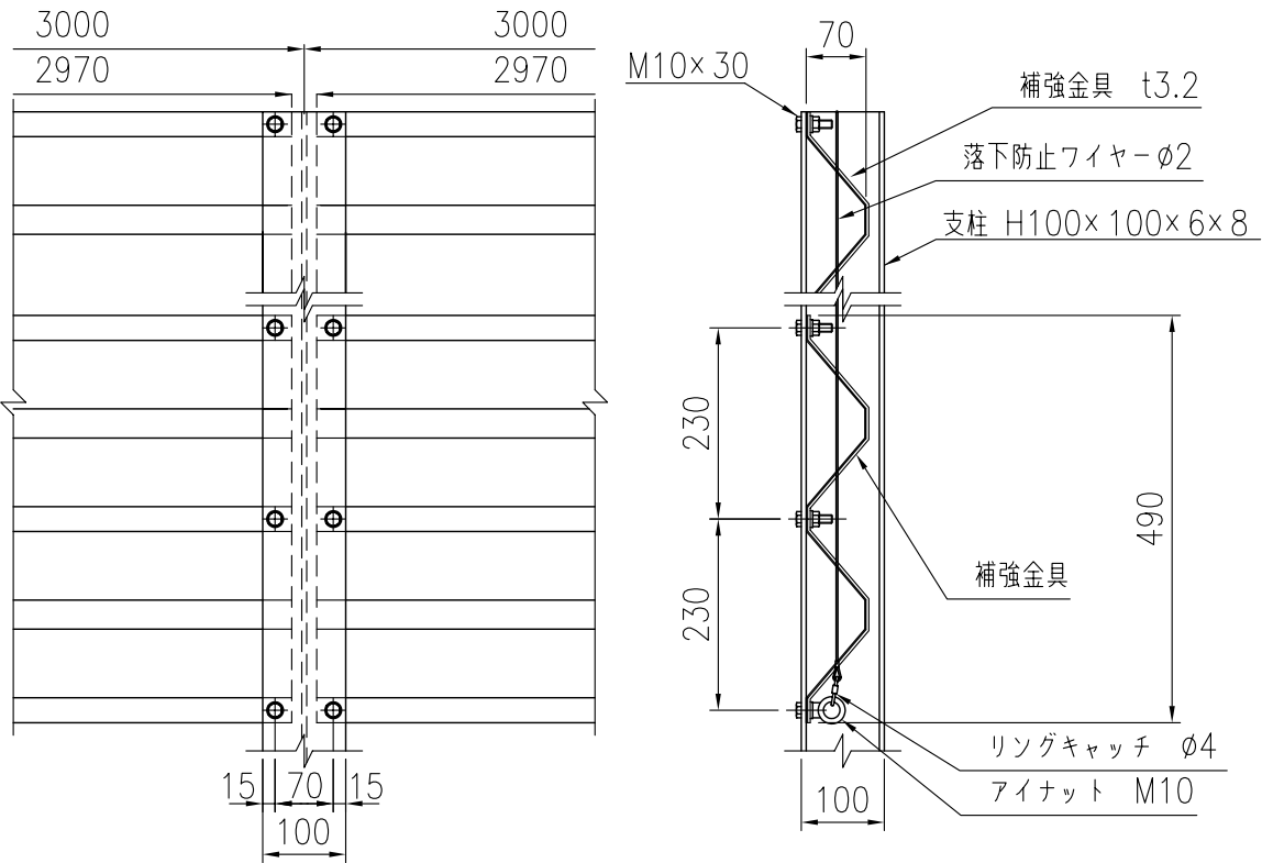
パンチングレール取付詳細図 (1/10)
