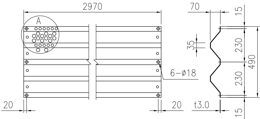
パンチングレール (1/15)
