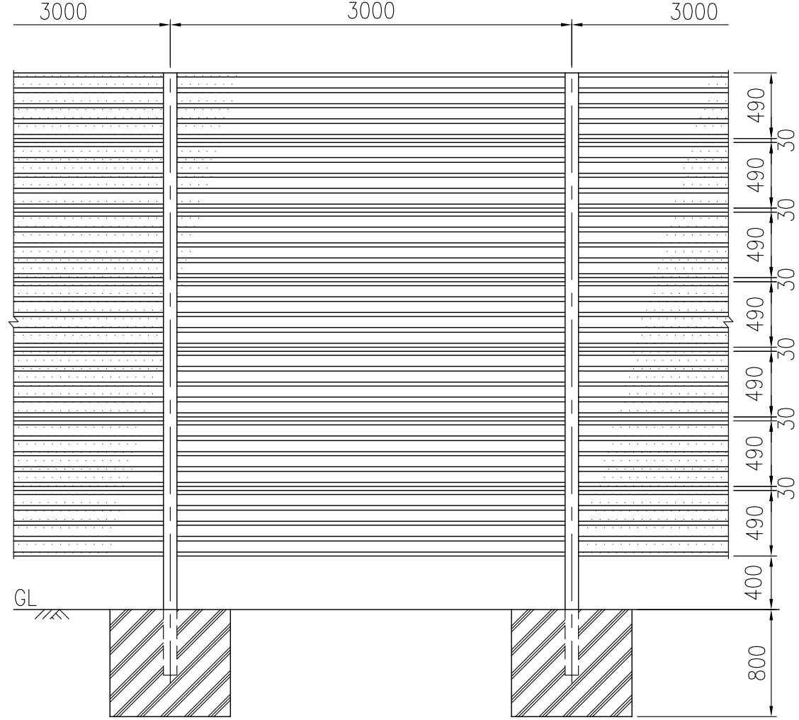
設置図 (1/40)
