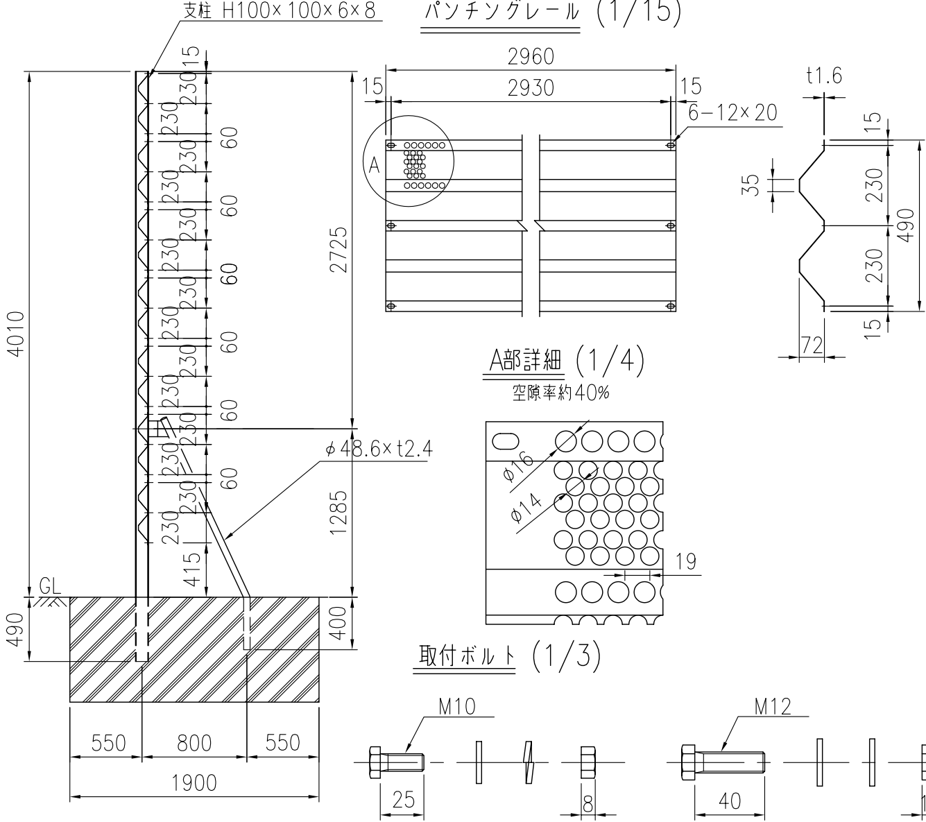
控柱取付詳細図 (1/10)
