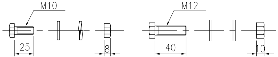
取付ボルト (1/3)
