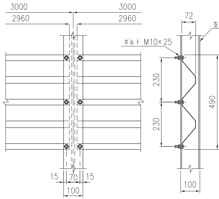
パンチングレール取付詳細図 (1/10)
