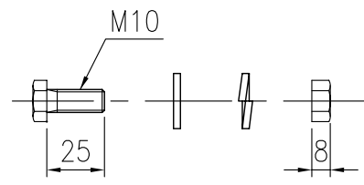
取付ボルト (1/3)
