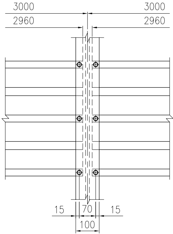
パンチングレール取付詳細図 (1/10)
