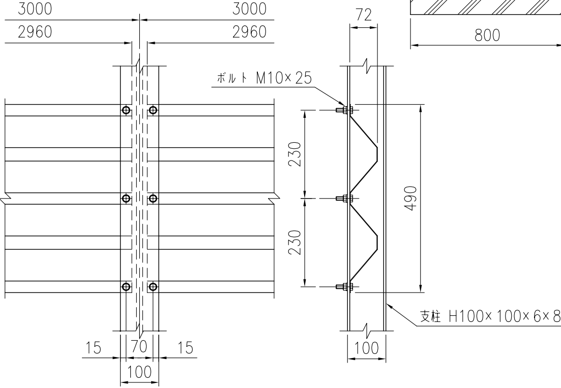
パンチングレール取付詳細図 (1/10)
