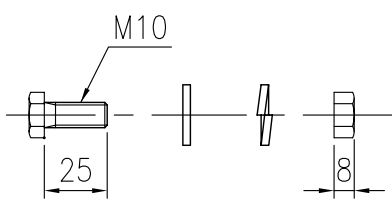
取付ボルト (1/3)
