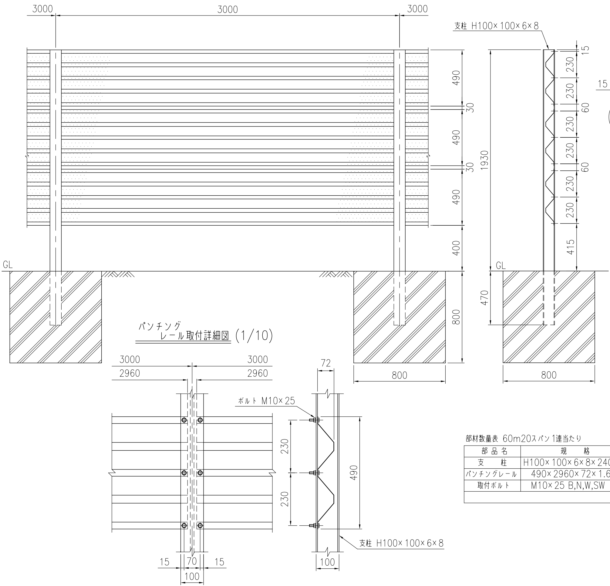
設置図 (1/20)
