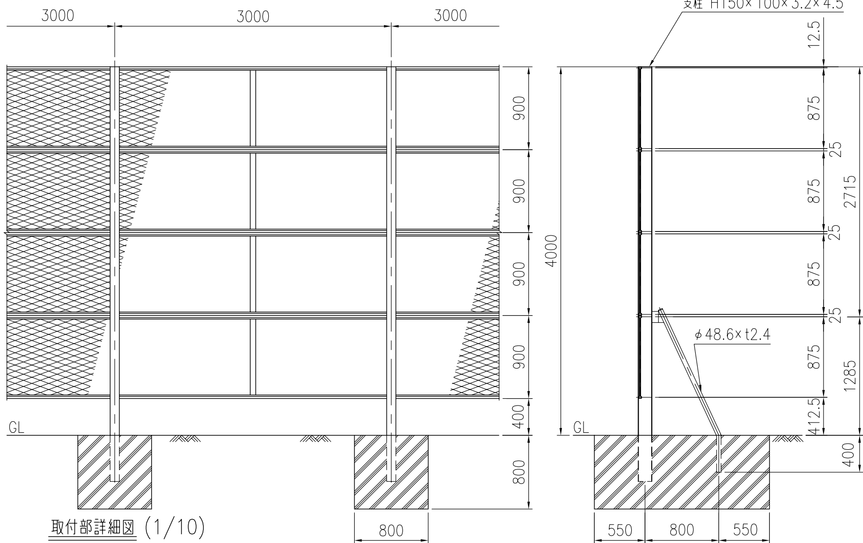
設置図 (1/40)
