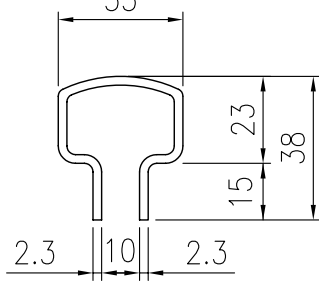
柵材断面 (1/2)
