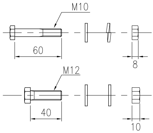
取付ボルト (1/3)
