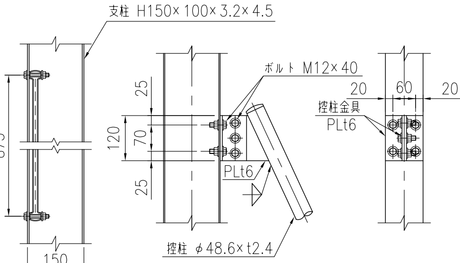
控柱取付詳細図 (1/10)
