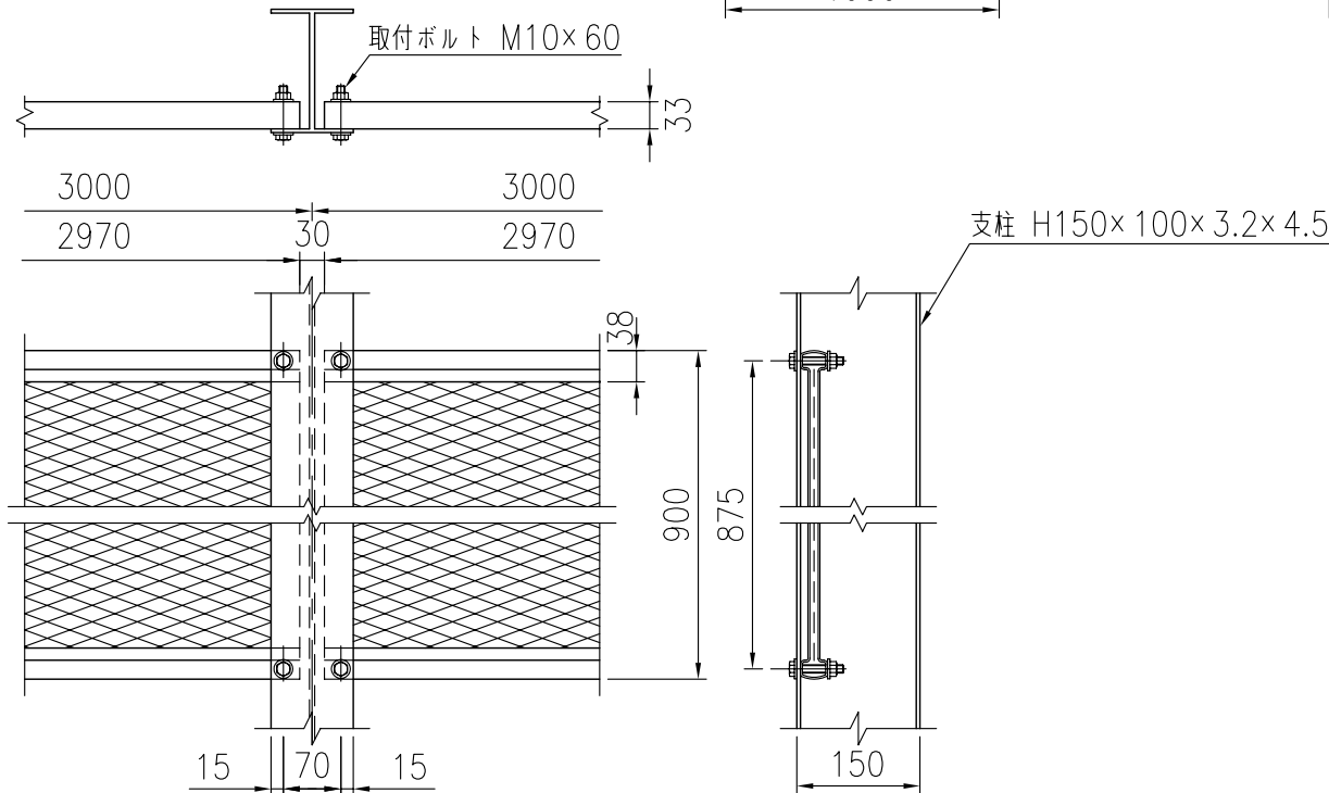
取付部詳細図 (1/10)
