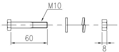
取付ボルト (1/3)
