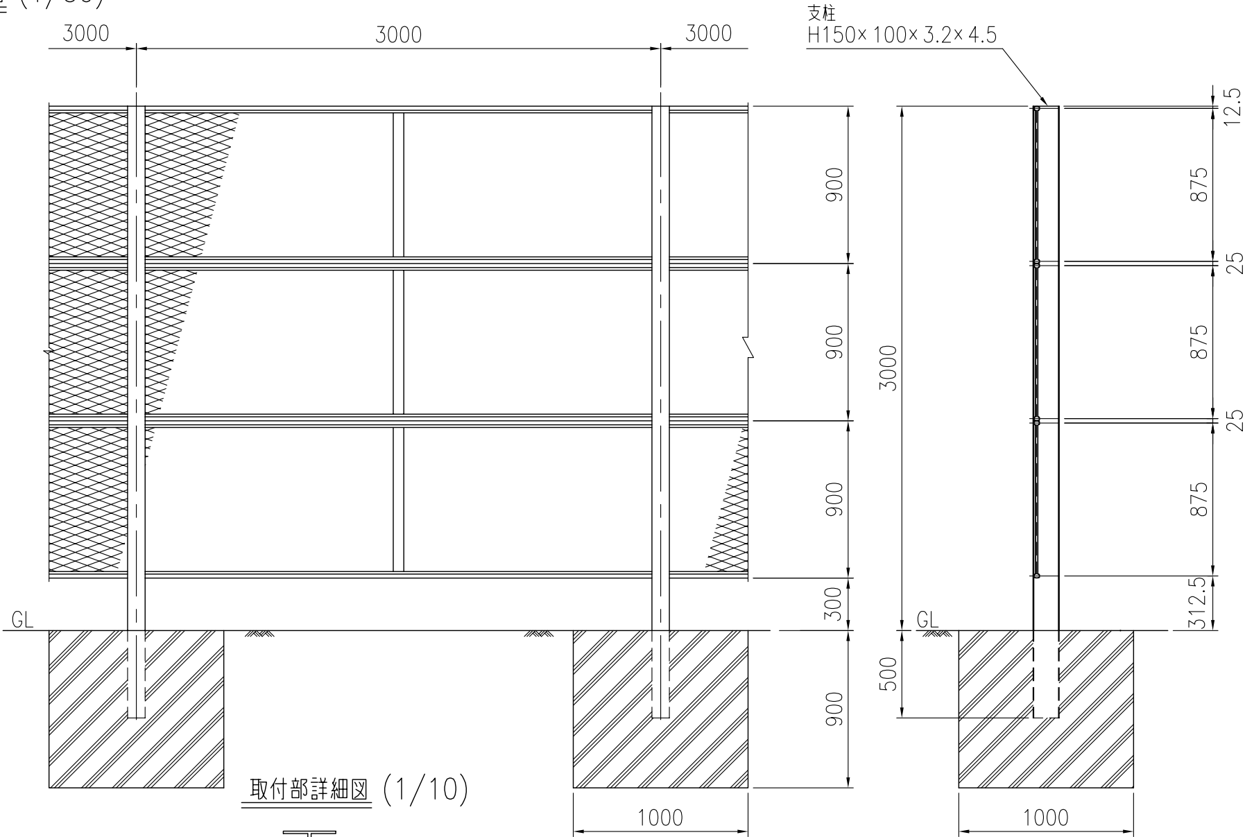
設置図 (1/30)
