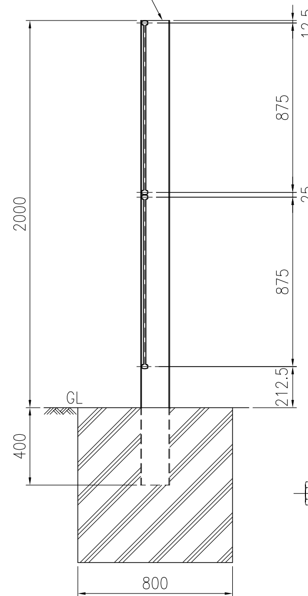
エキスパンドメタル (1/2)
