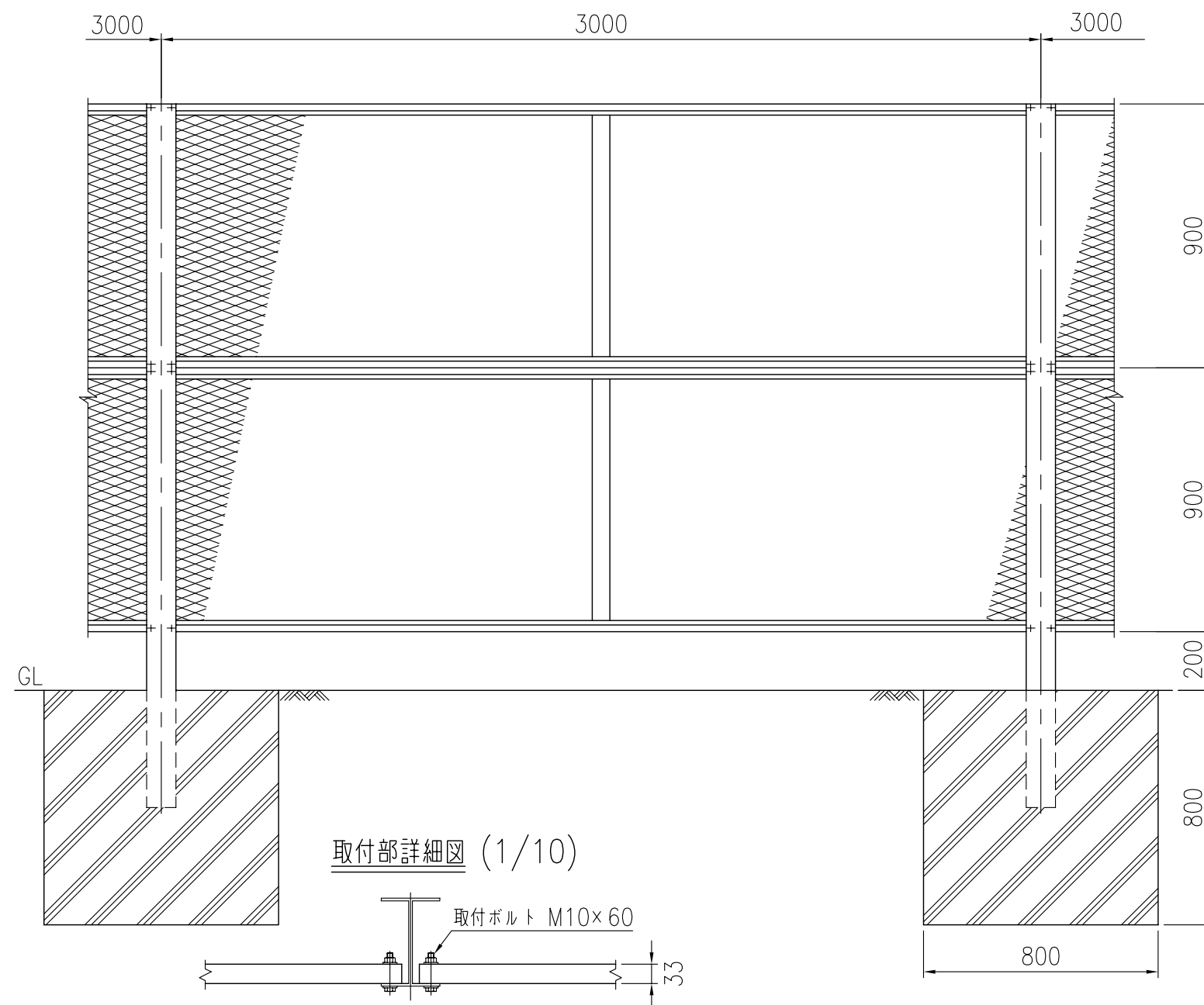
設置図 (1/20)
