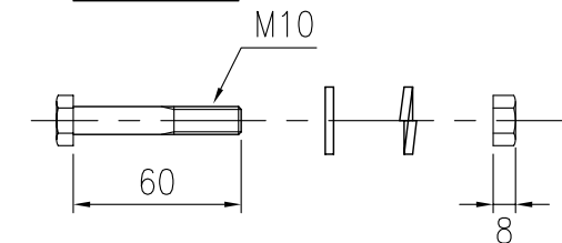
取付ボルト (1/3)
