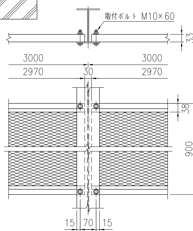
取付部詳細図 (1/10)
