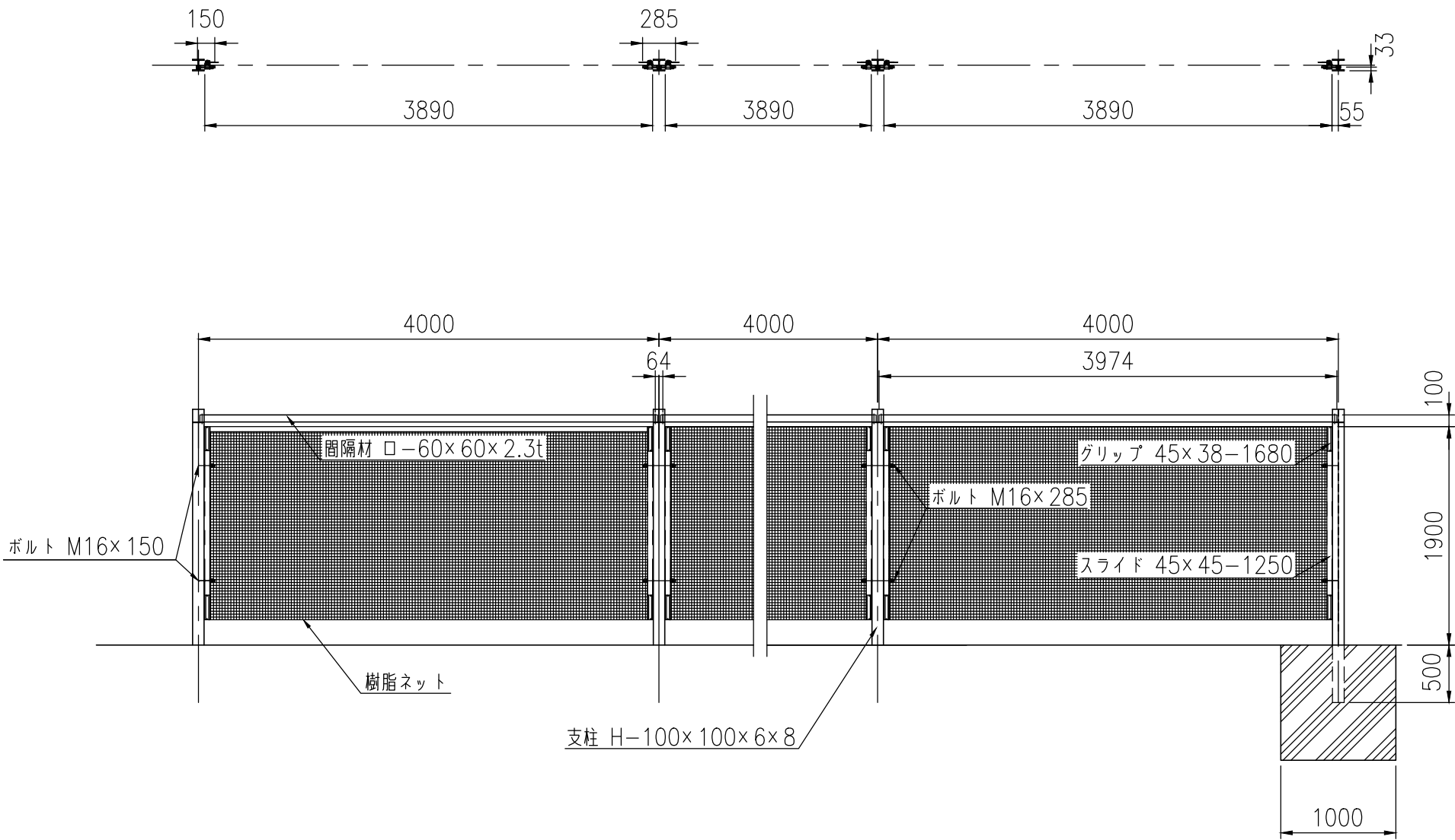
設置正面図
