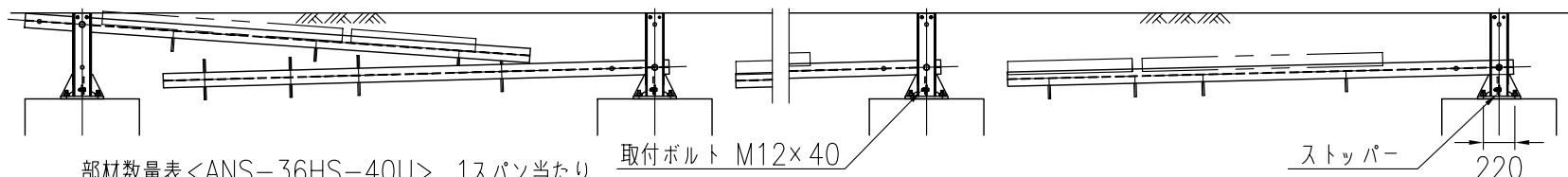
部材数量表<ANS-36HS-40U> 1スパン当たり
