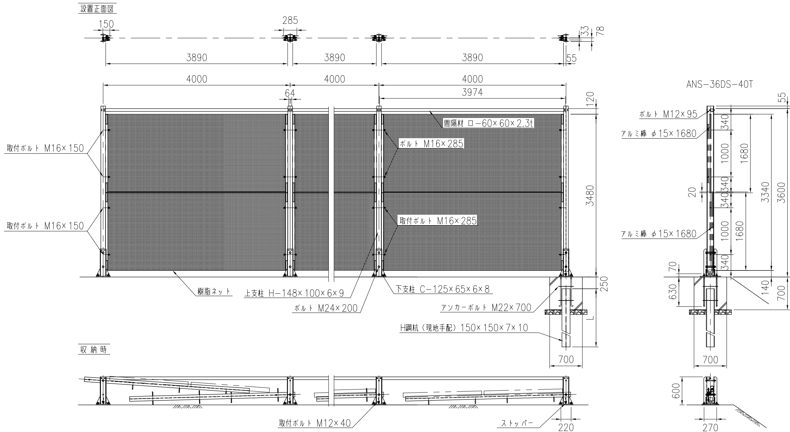
部材数量表<ANS-36DS-40T> 1スパン当たり
