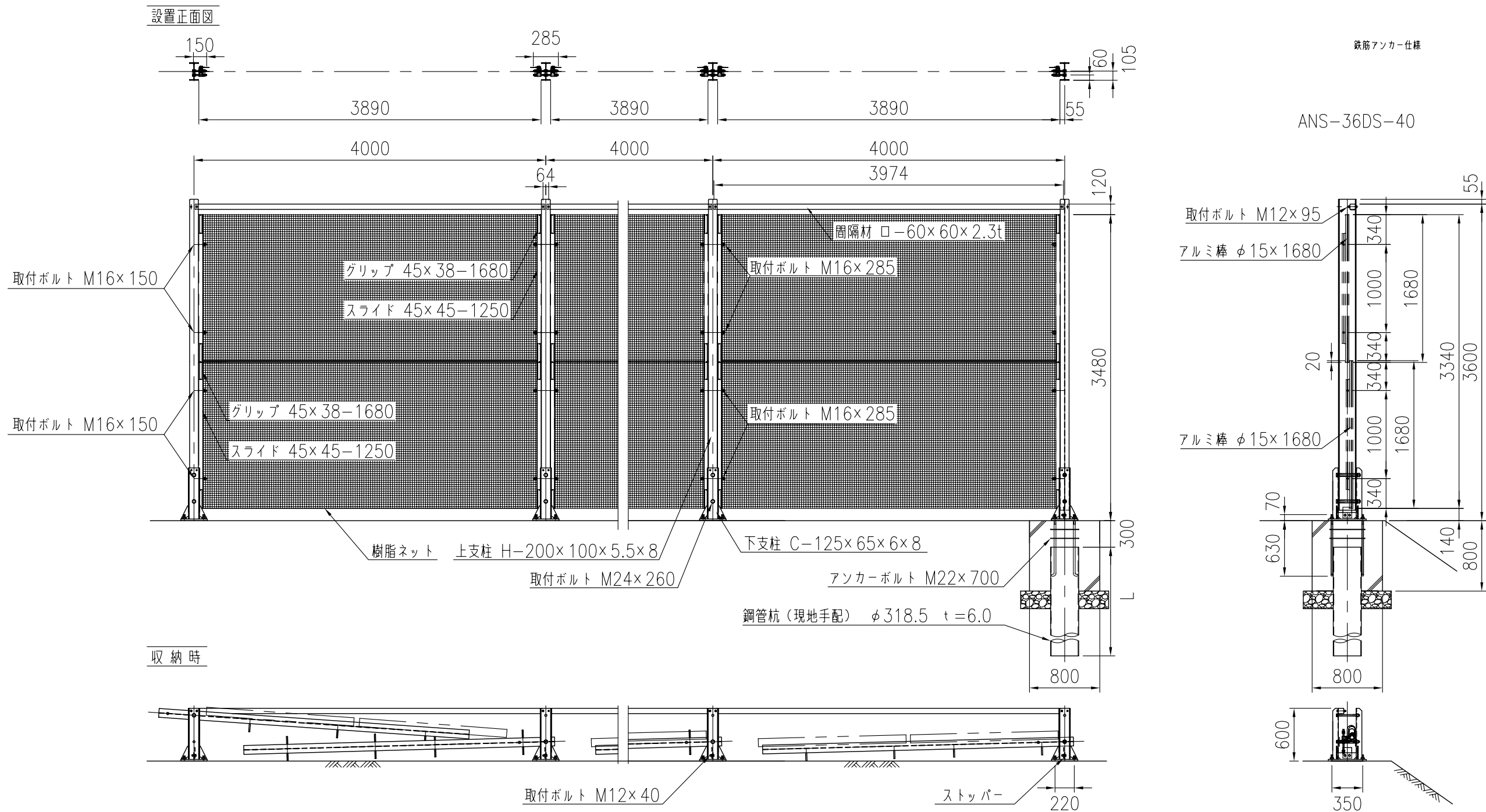
部材数量表<ANS-36DS-40> 1スパン当たり
