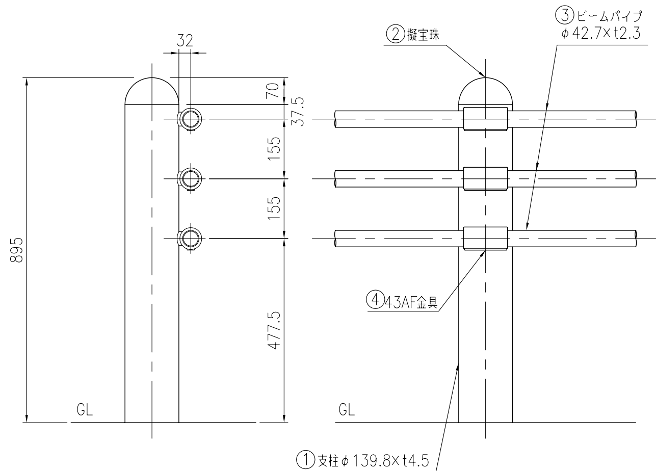
支柱図
