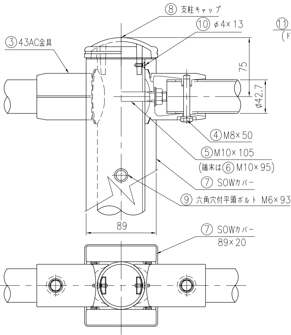
取付部詳細図 (1/3)
