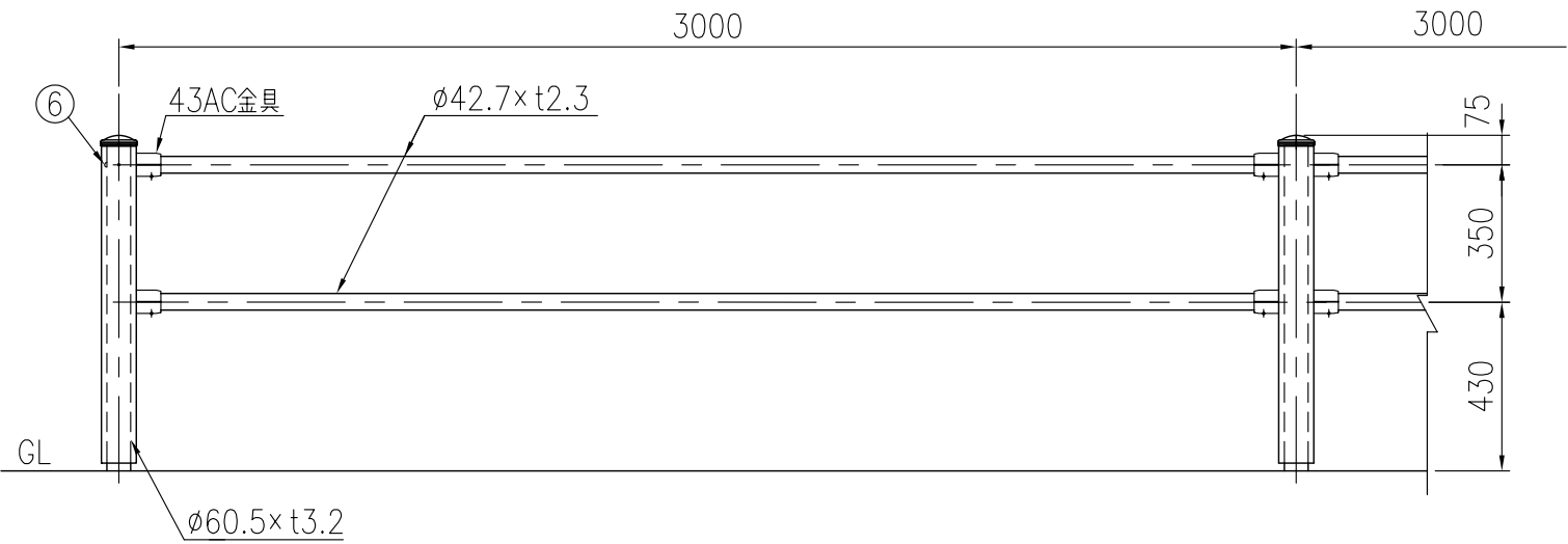
設置図 (1/20)
