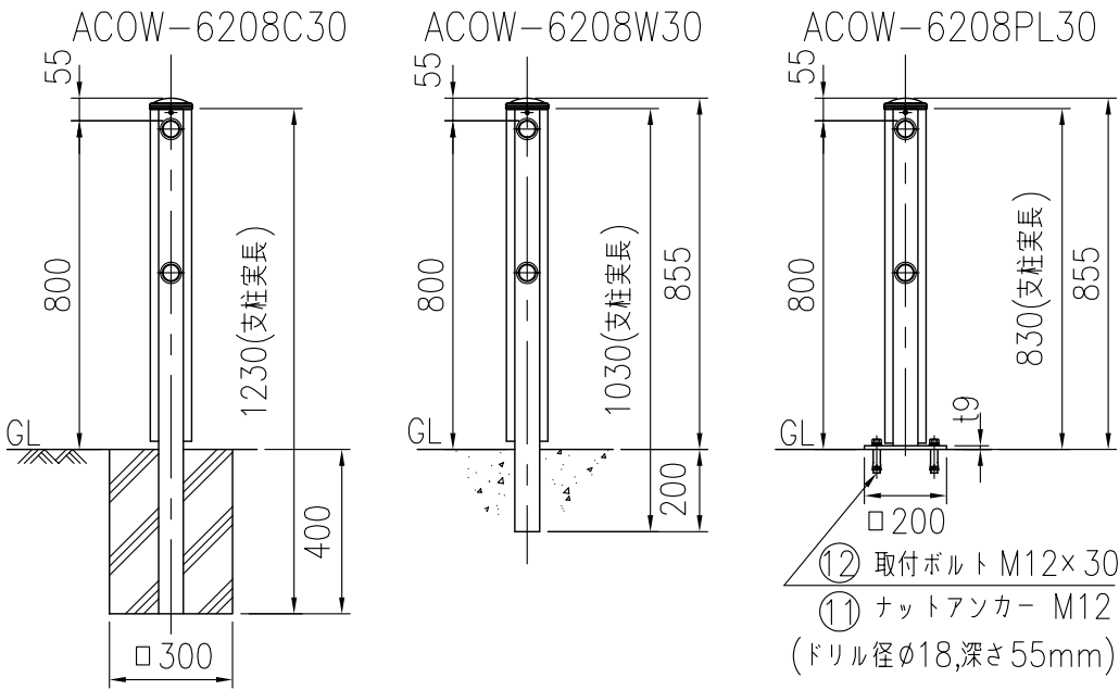
ベースプレート詳細図 (1/10)
