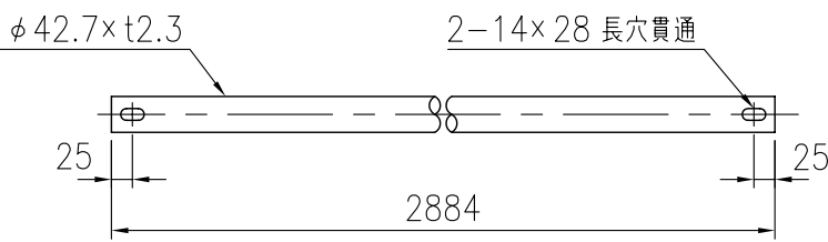
ビーム図 (1/10)
