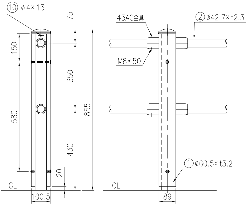
支柱図 (1/10)
