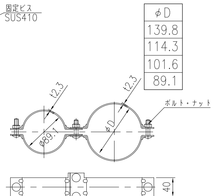
親子バンド詳細図 S=1/5
