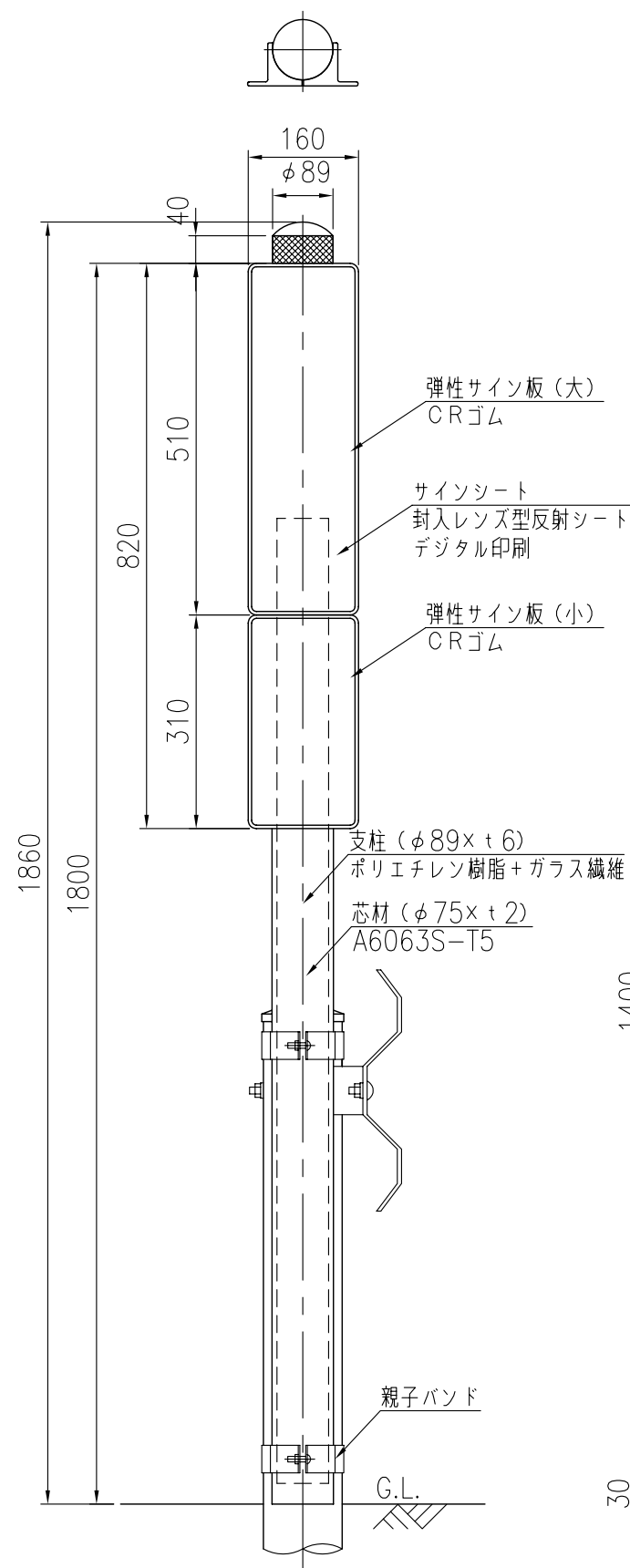
設置図 S=1/10
