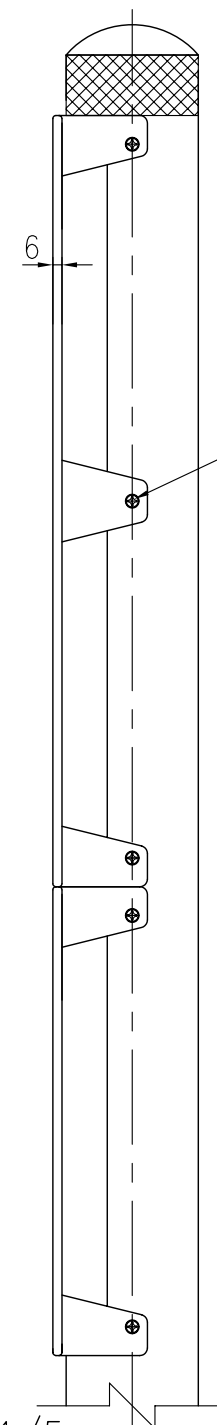
標示部詳細 S=1/5
