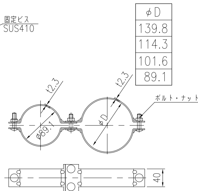
親子バンド詳細図 S=1/5
