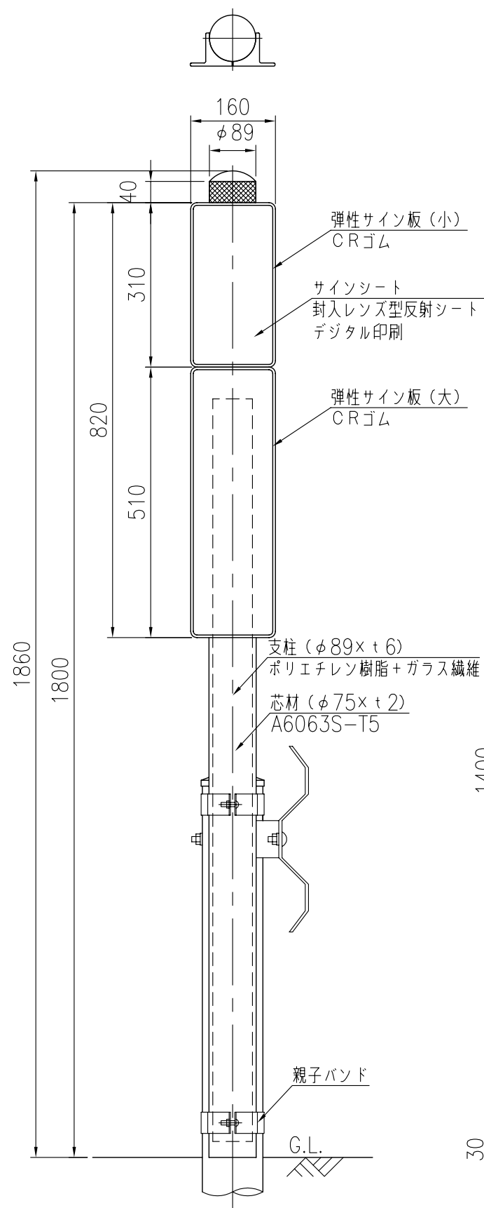
設置図 S=1/10
