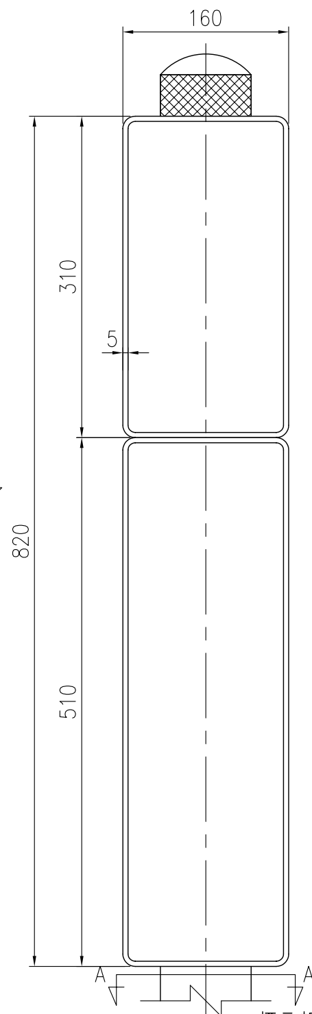
標示部詳細 S=1/5
