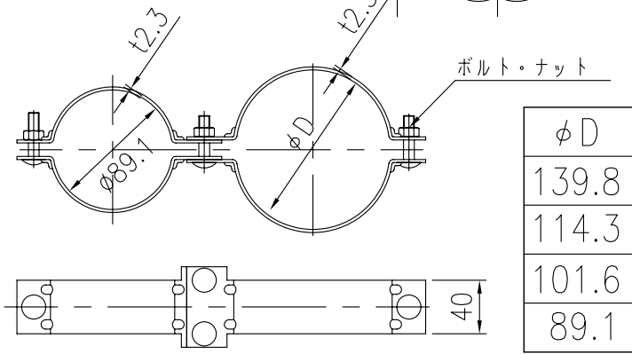
親子バンド詳細図 S=1/5
