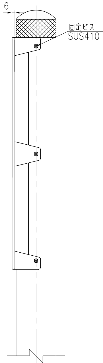
標示部詳細 S=1/5
