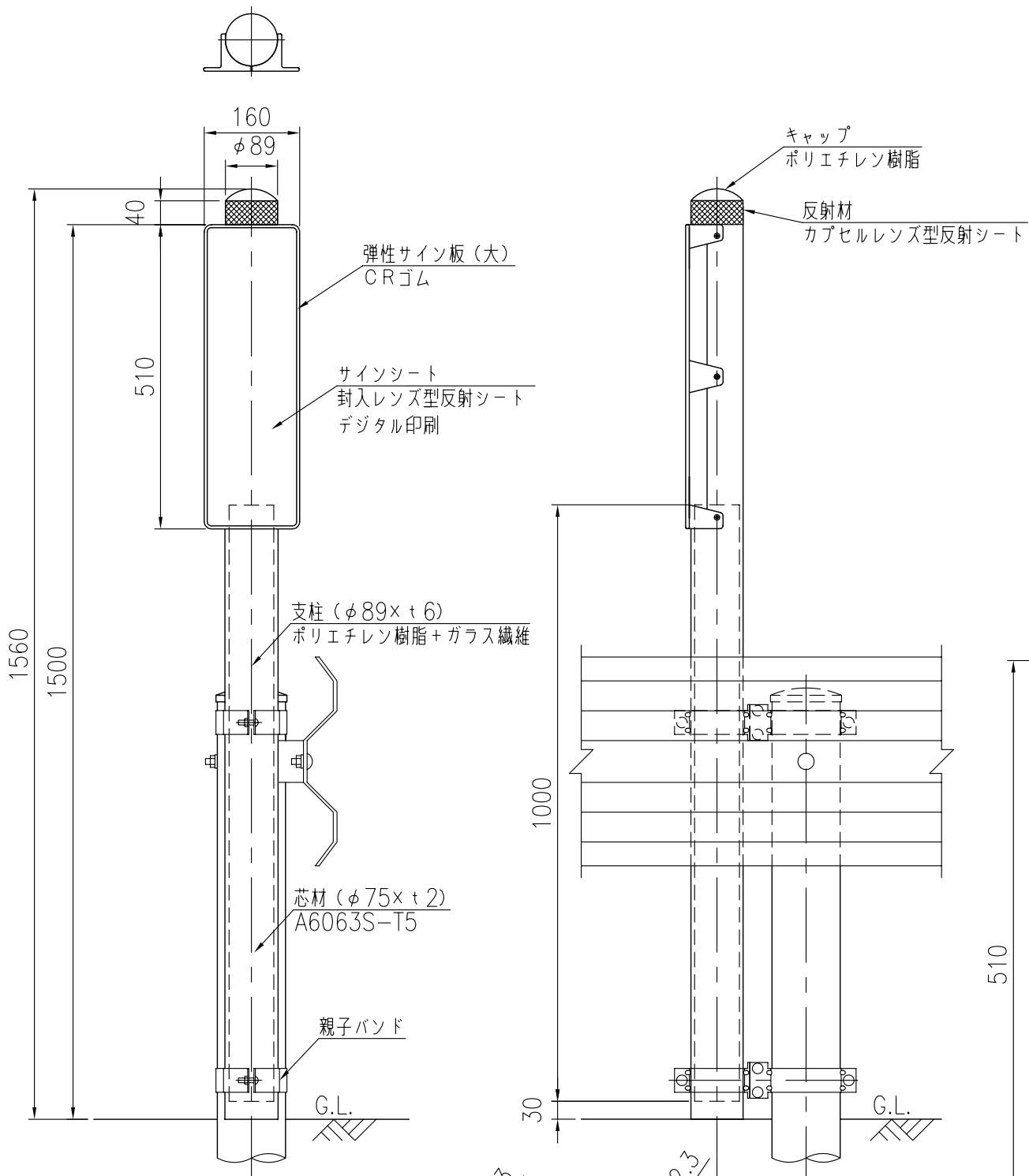
設置図 S=1/10
