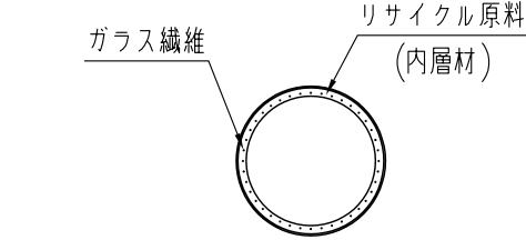
A-A 断面図 S=1/5
