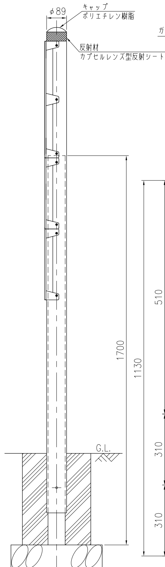
設置図 S=1/10
