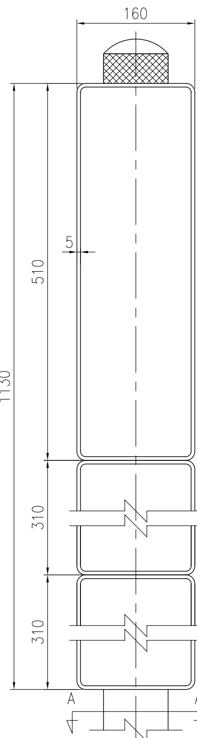
標示部詳細 S=1/5
