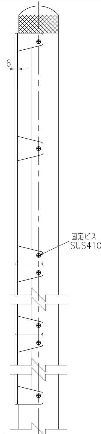
標示部詳細 S=1/5
