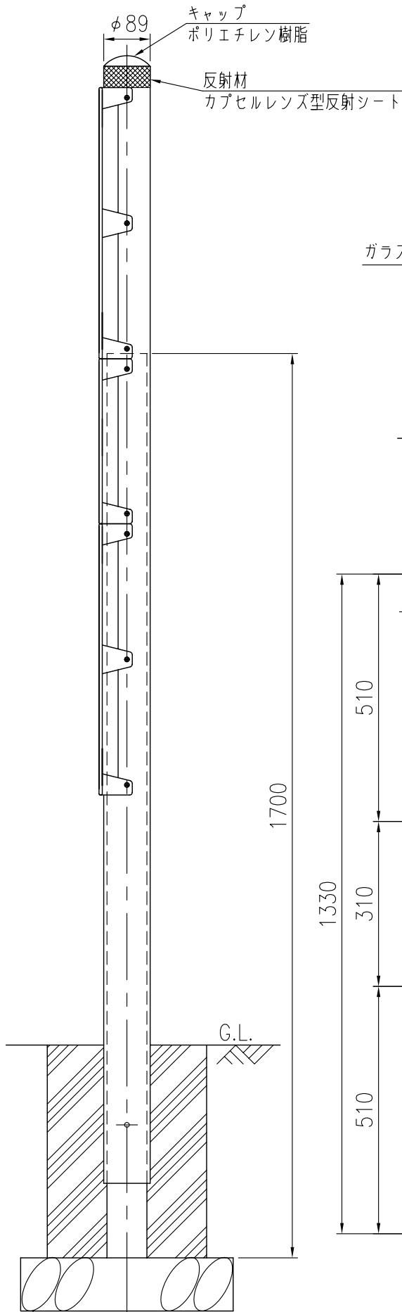
設置図 S=1/10
