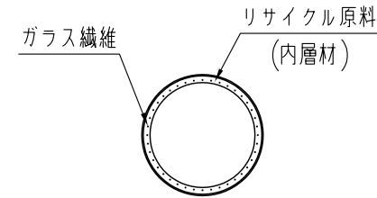
A-A 断面図 S=1/5
