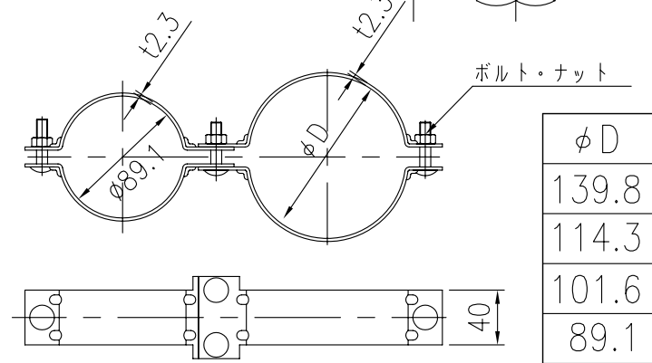
親子バンド詳細図 S=1/5
