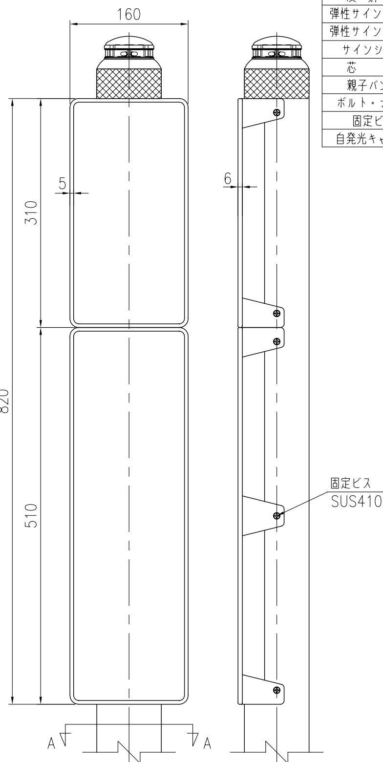
標示部詳細 S=1/5
