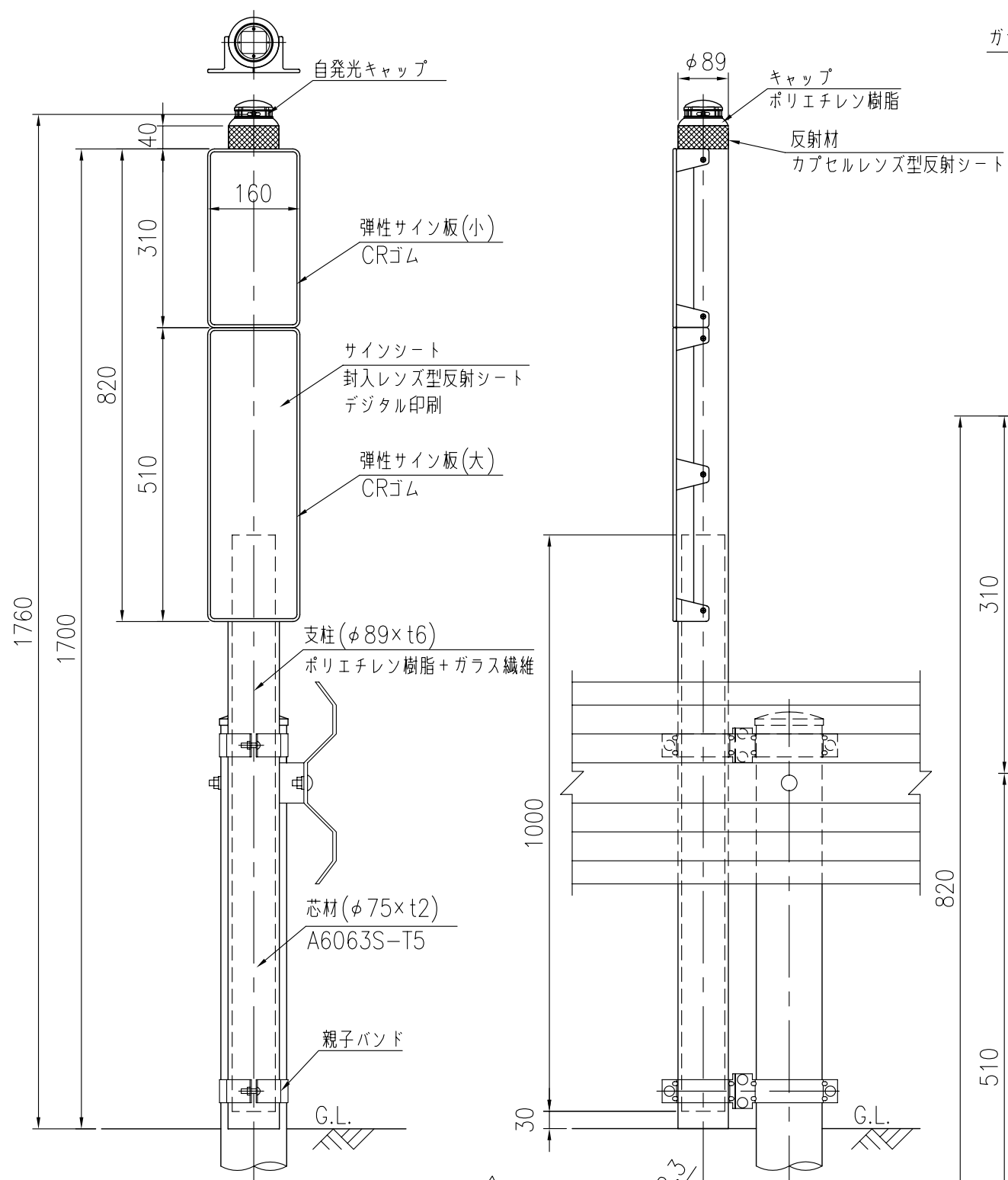
設置図 S=1/10
