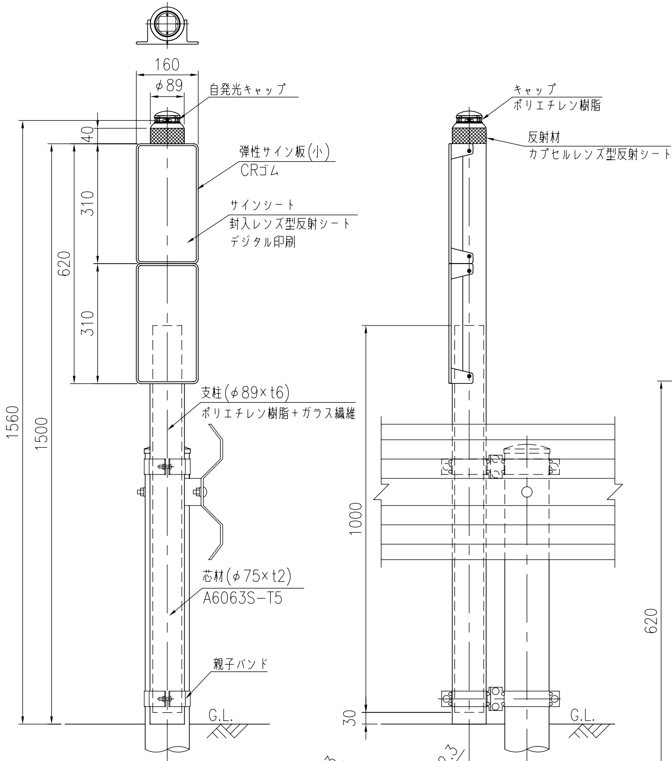
設置図 S=1/10
