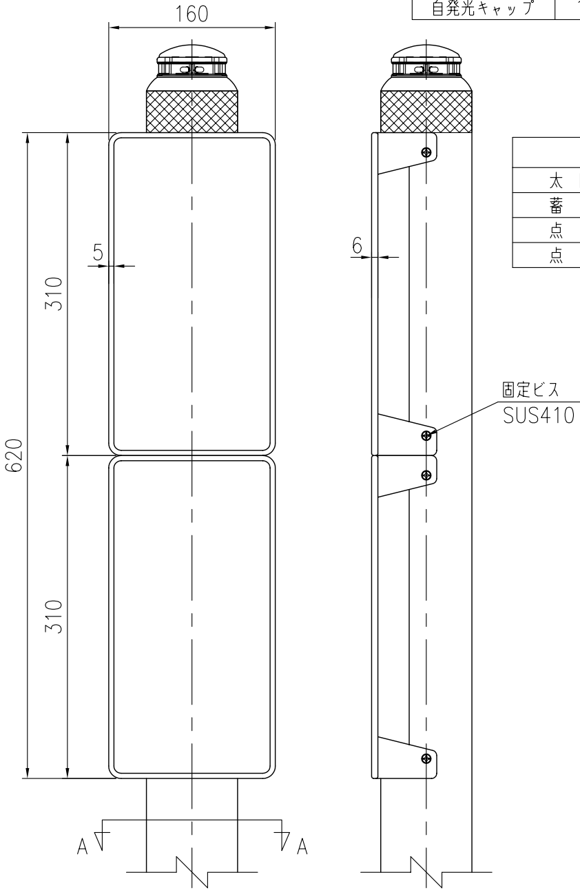
標示部詳細 S=1/5
