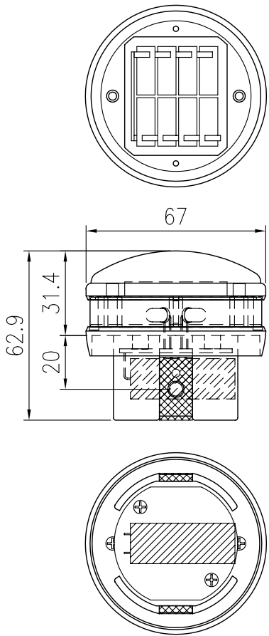
SLキャップ80 S=1/2
