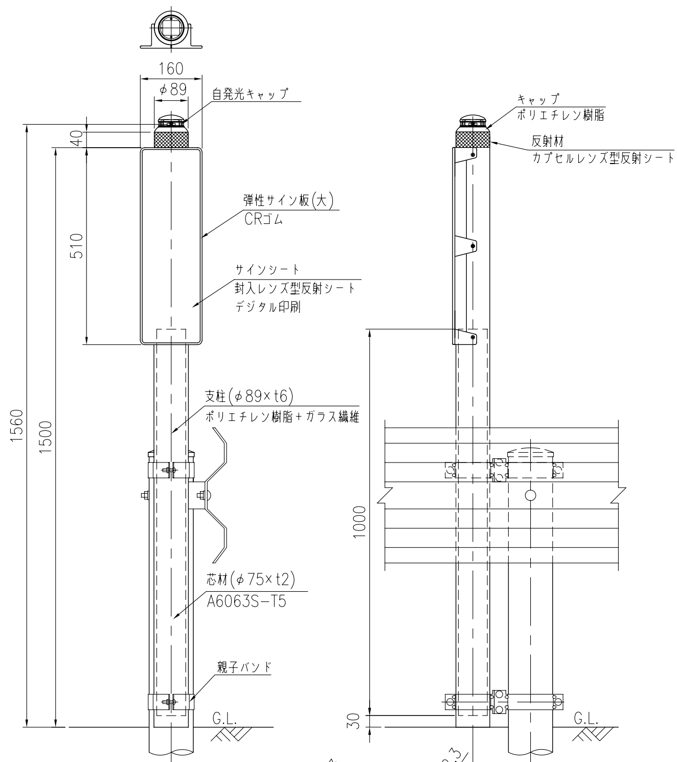
設置図 S=1/10
