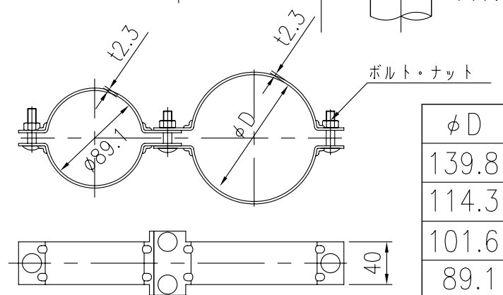
親子バンド詳細図 S=1/5
