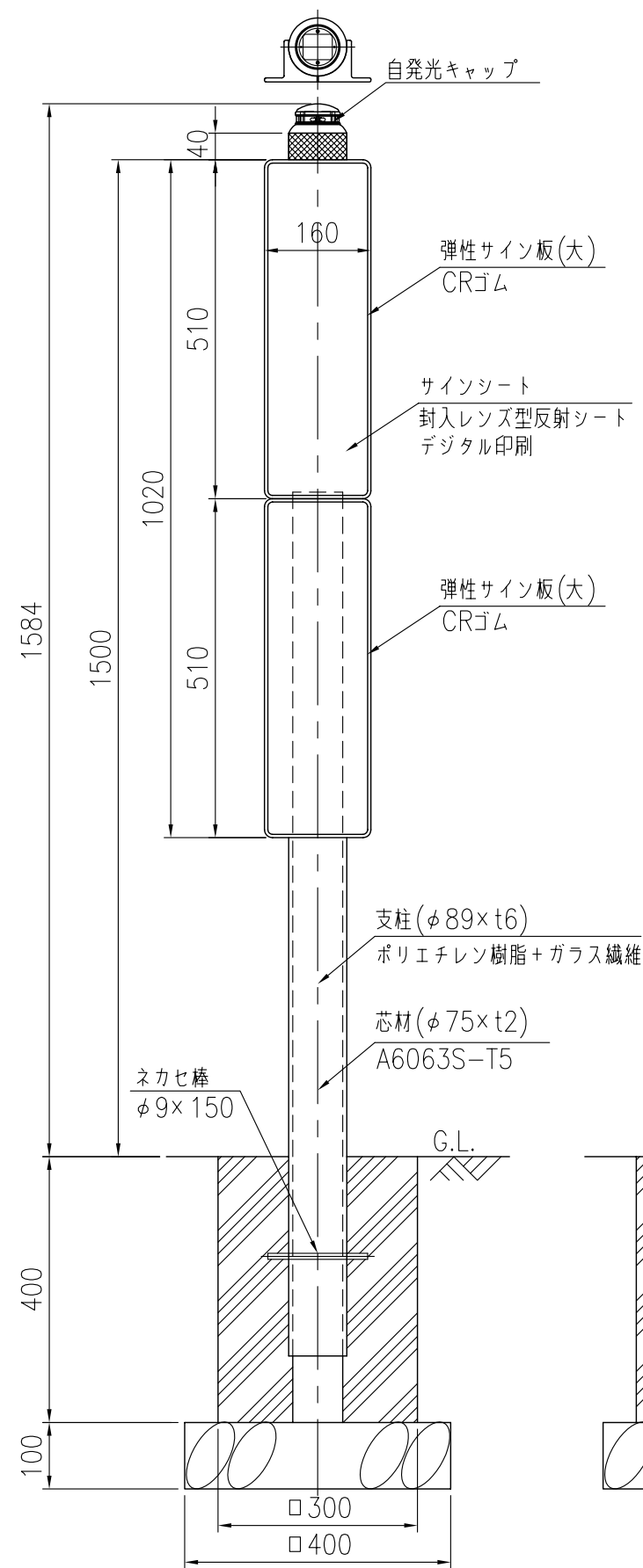
設置図 S=1/10
