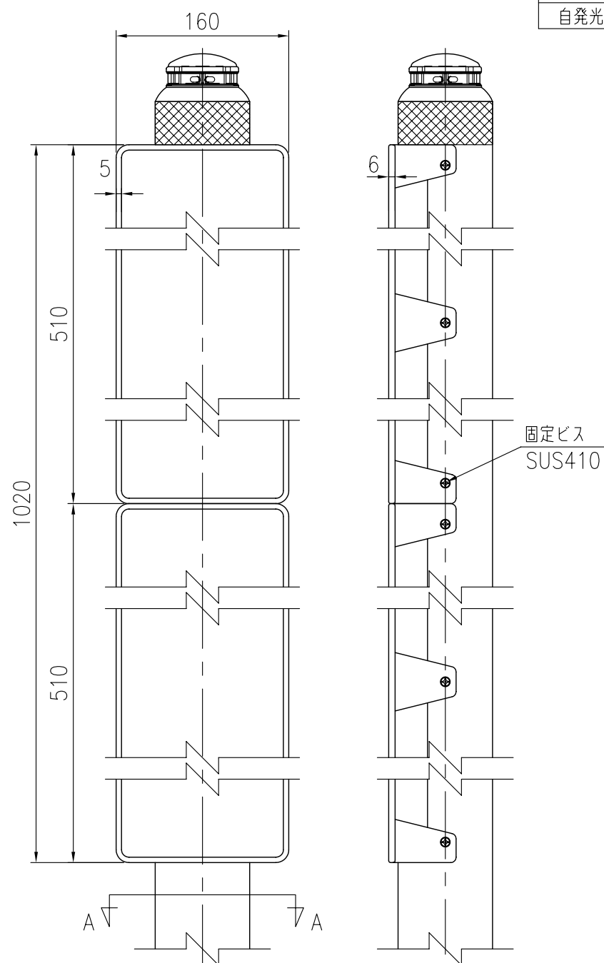
標示部詳細 S=1/5
