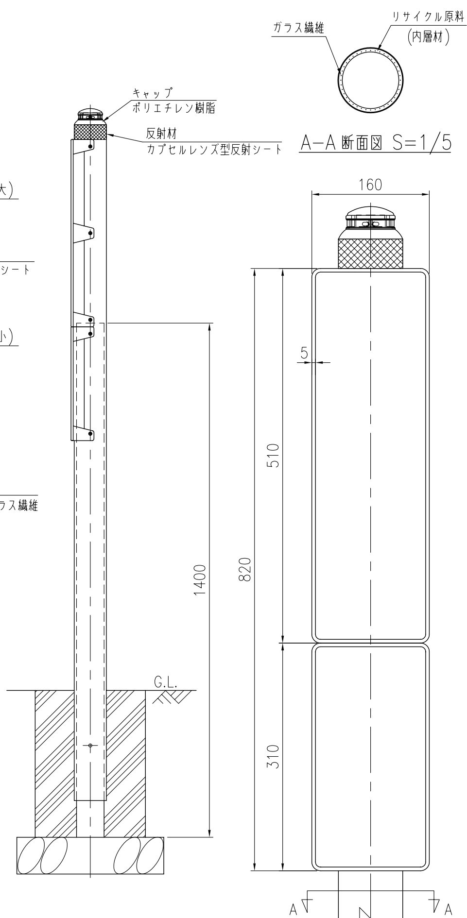
標示部詳細 S=1/5
