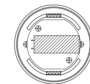
SLキャップ80 S=1/2
