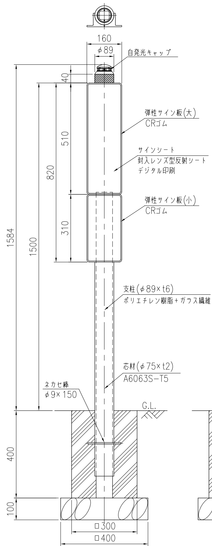
設置図 S=1/10
