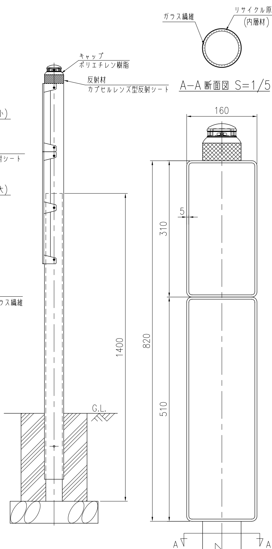
標示部詳細 S=1/5
