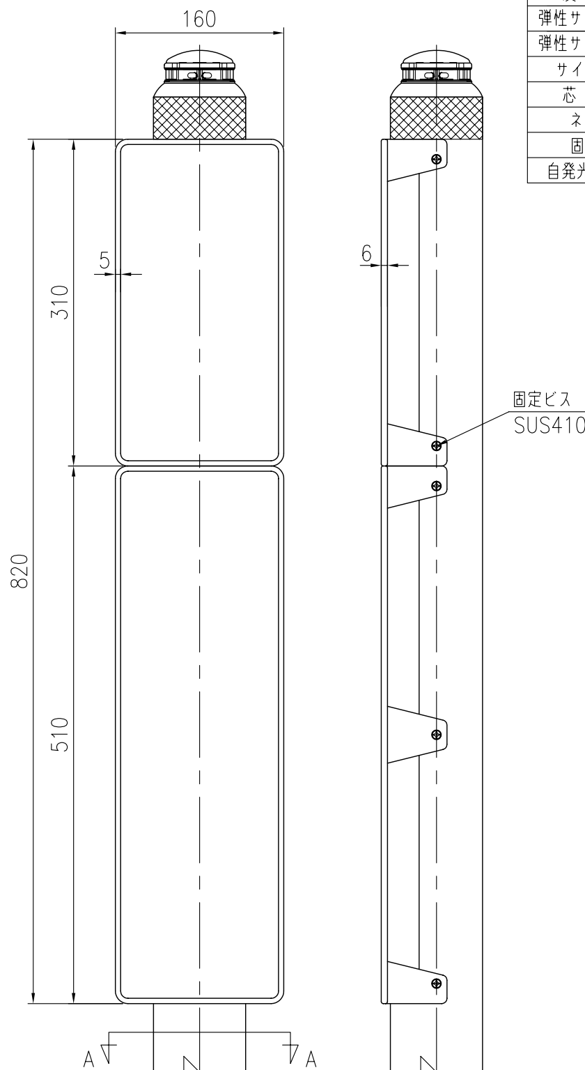
標示部詳細 S=1/5
