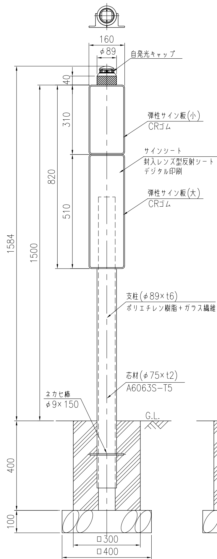
設置図 S=1/10
