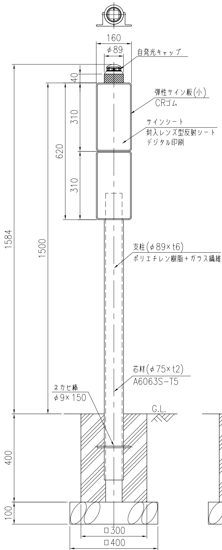
設置図 S=1/10
