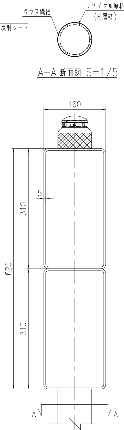
標示部詳細 S=1/5
