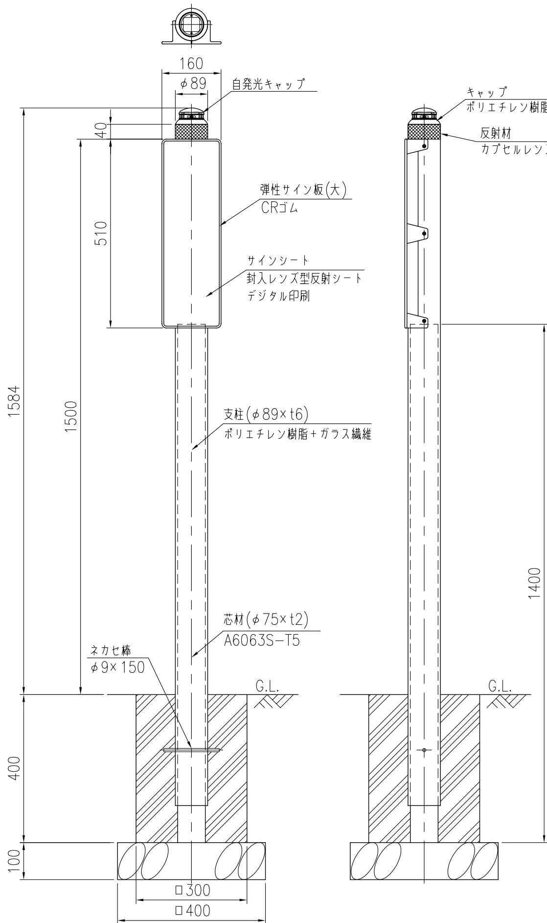
設置図 S=1/10
