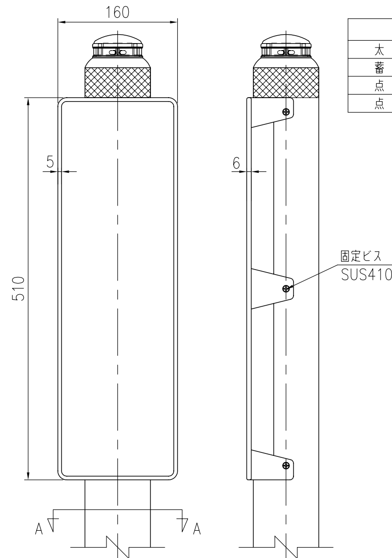
標示部詳細 S=1/5
