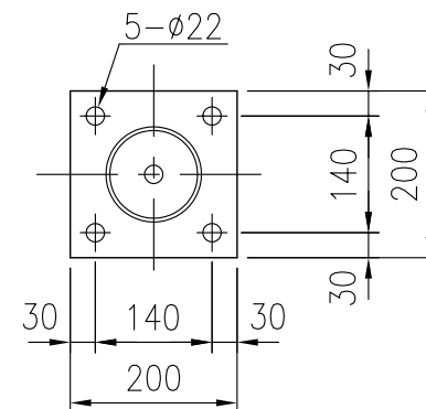
ベースプレート詳細図 (1/10)
