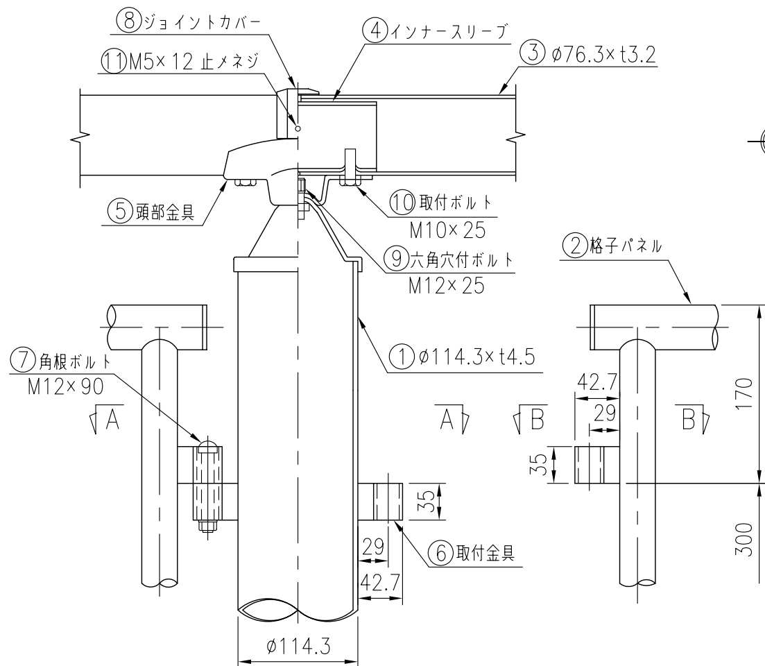
取付部詳細図 (1/5)
