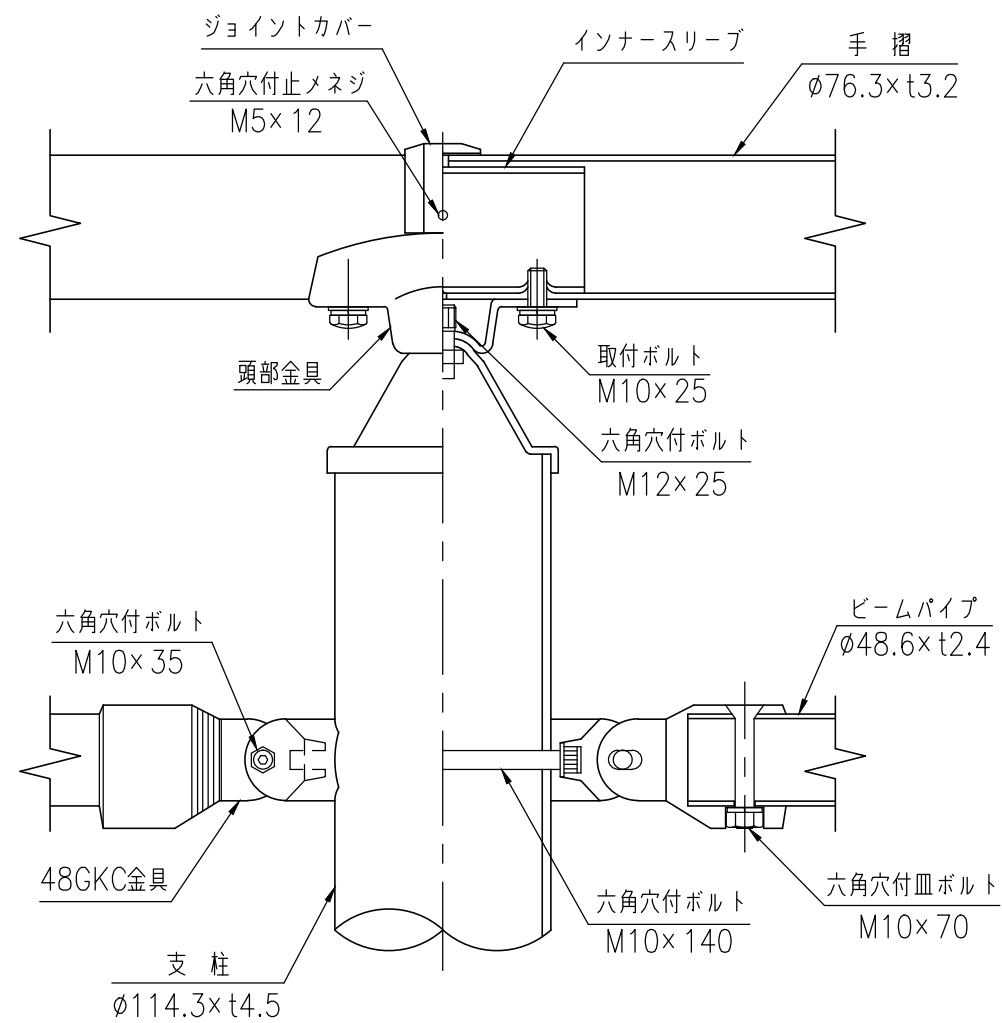
取付部詳細図 (1/4)
