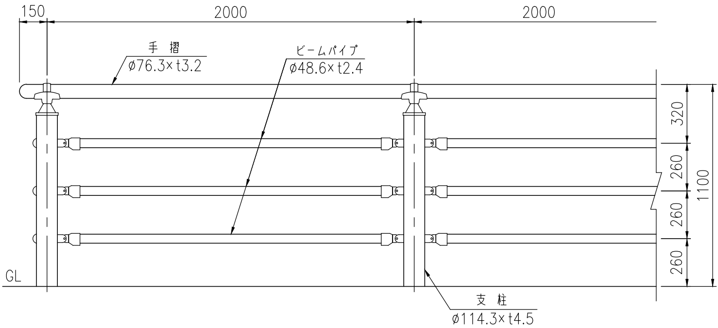
設置図 (1/20)
