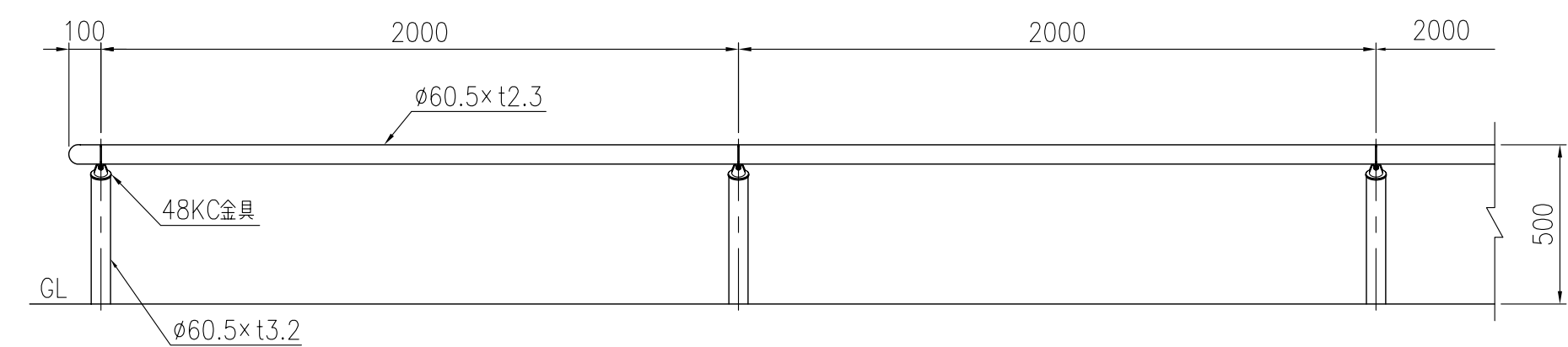
設置図 (1/20)
