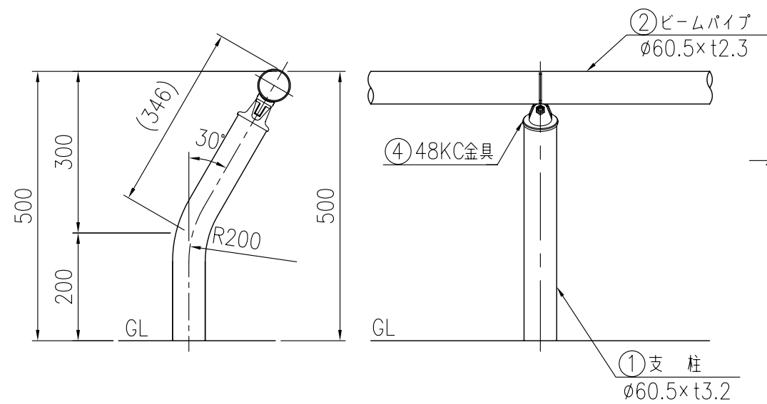
支柱図 (1/10)
