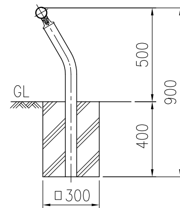
61KC-6105C20 (曲柱仕様)
