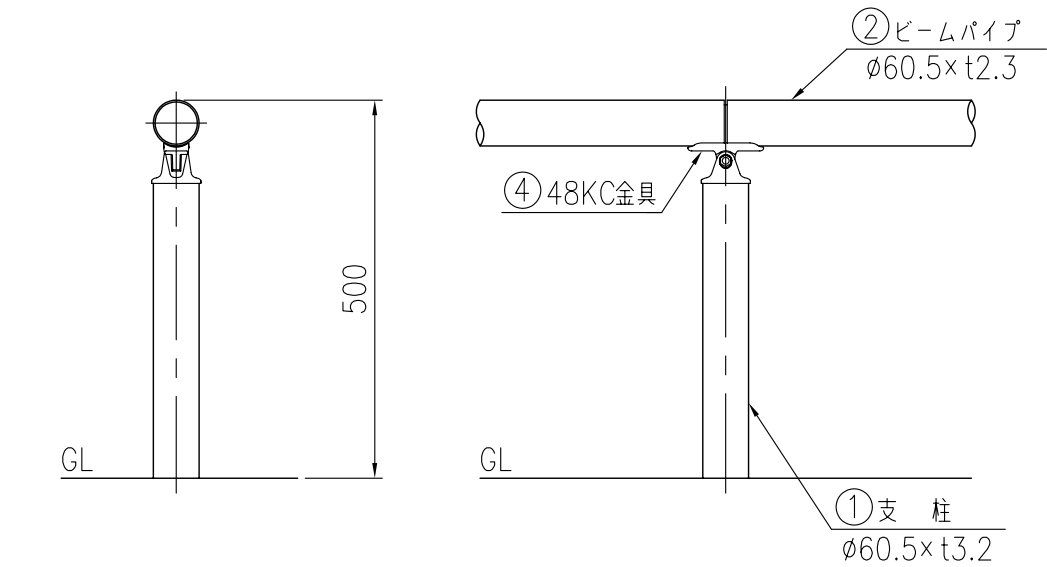
支柱図 (1/10)
