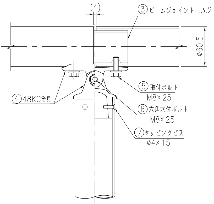
取付部詳細図 (1/3)
