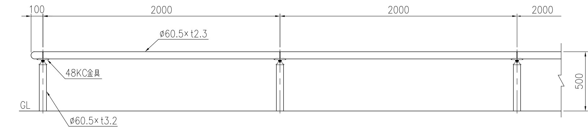
設置図 (1/20)
