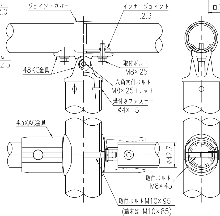
取付部詳細図 (1/3)
