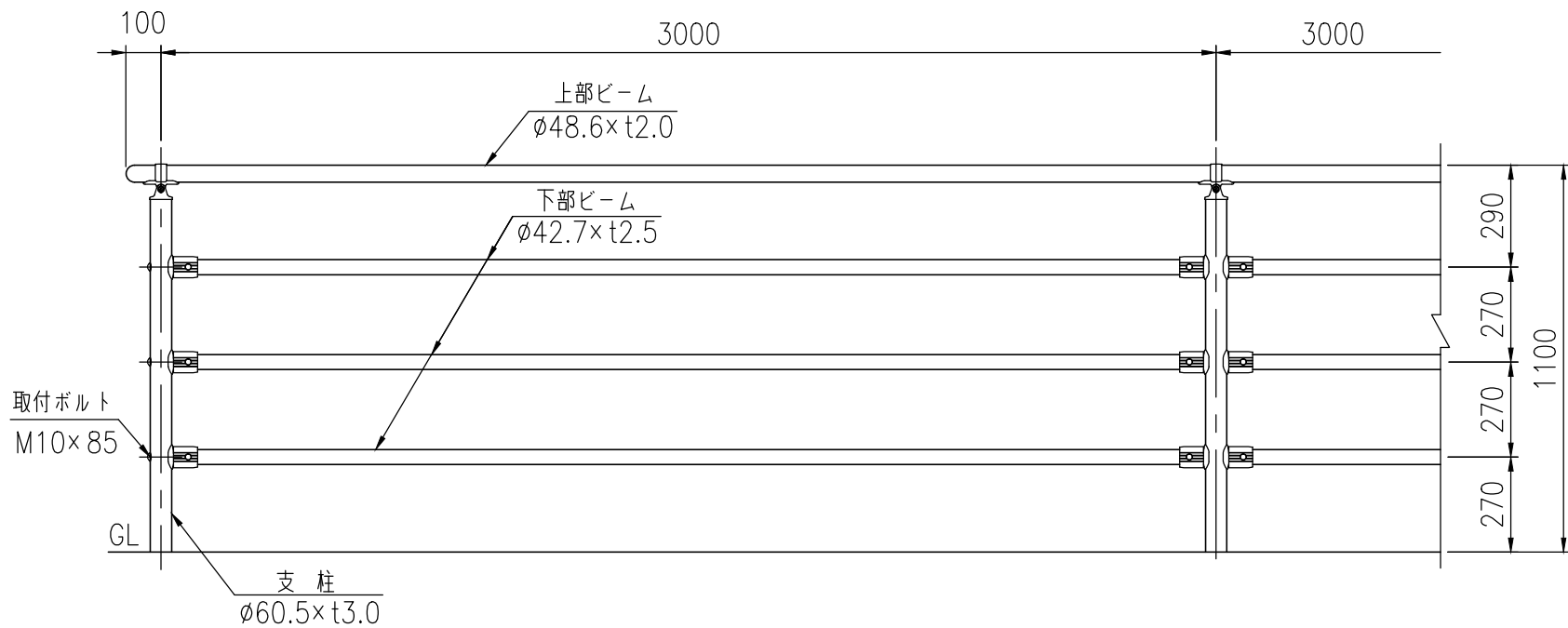
取付部詳細図 (1/3)
