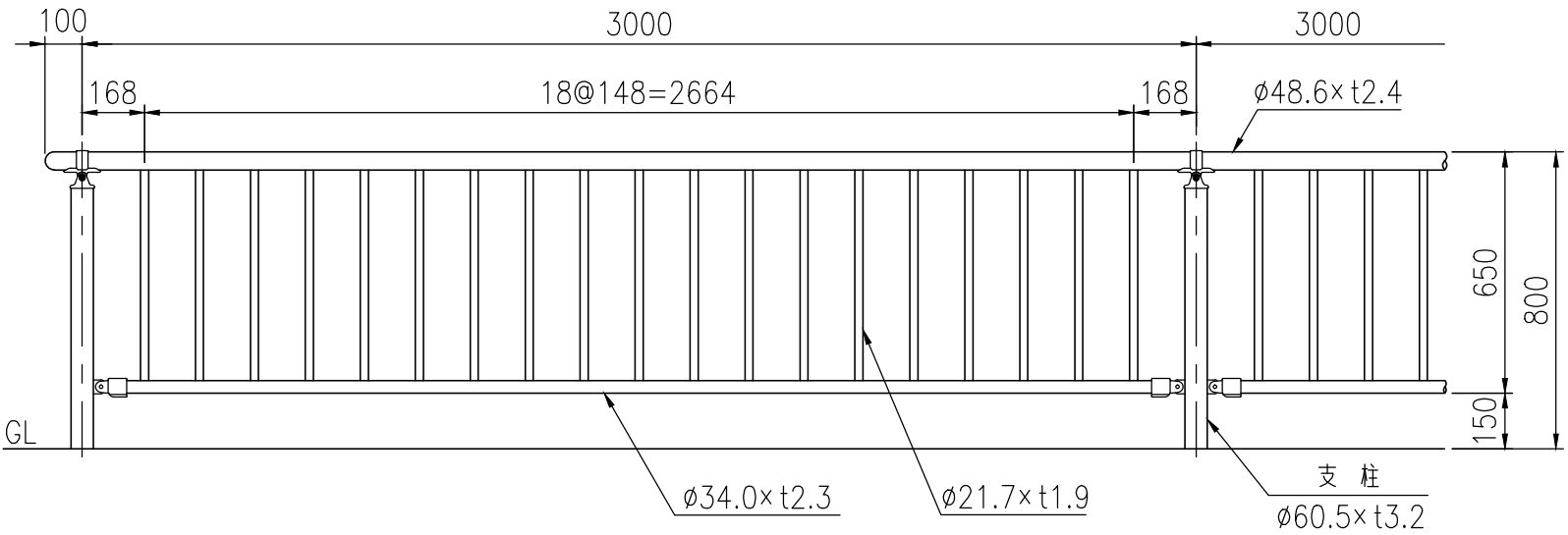
設置図 (1/20)
