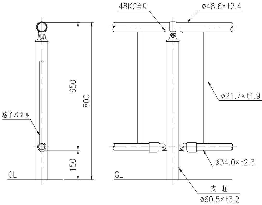
支柱図 (1/10)
