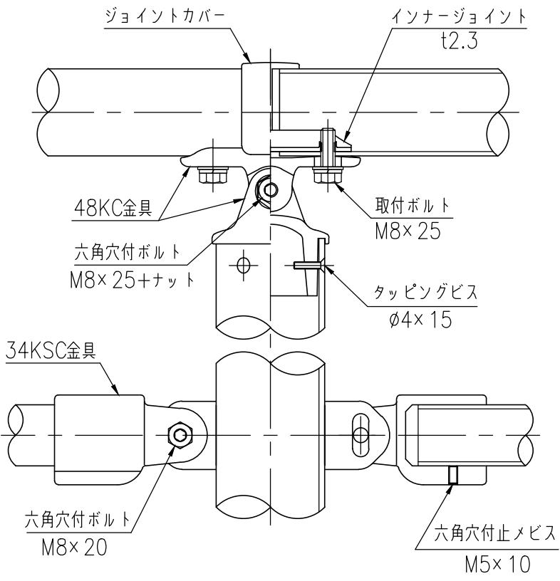
取付部詳細図 (1/3)
