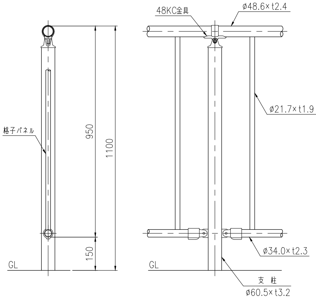
支柱図 (1/10)
