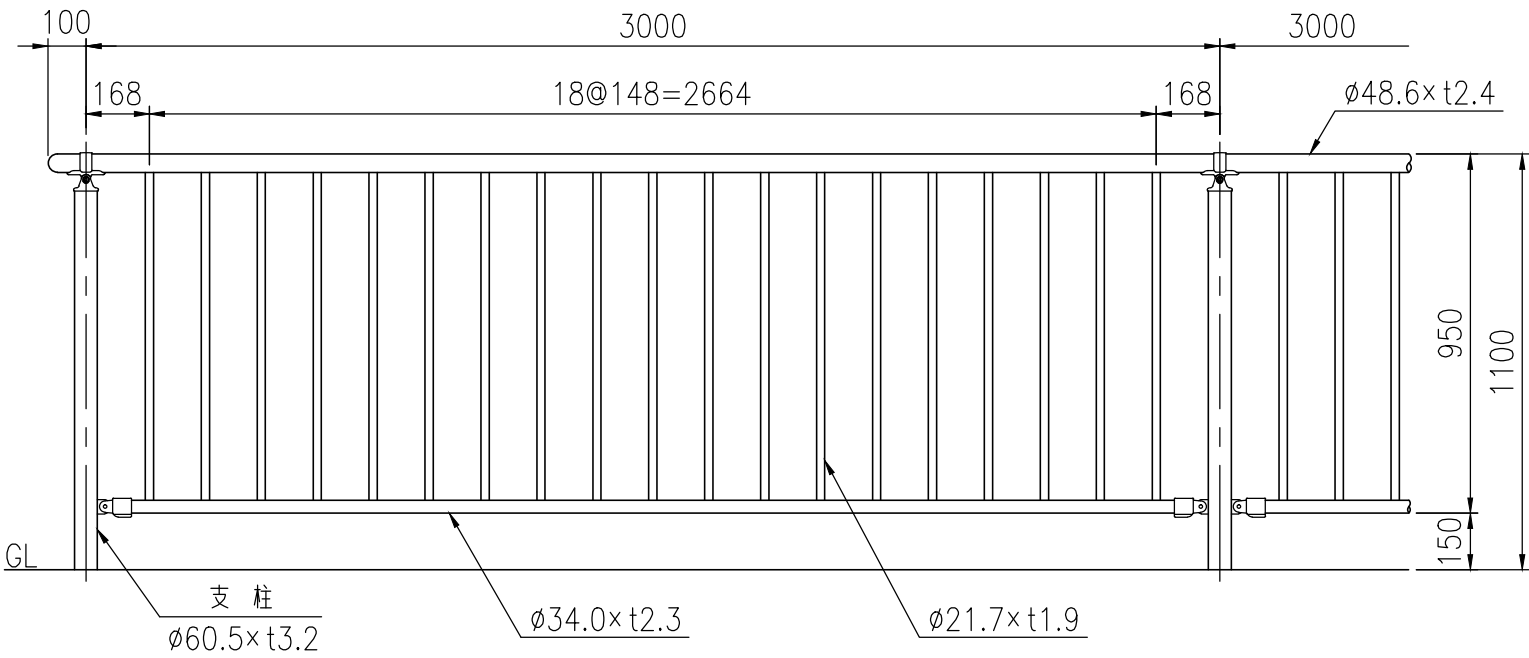
設置図 (1/20)
