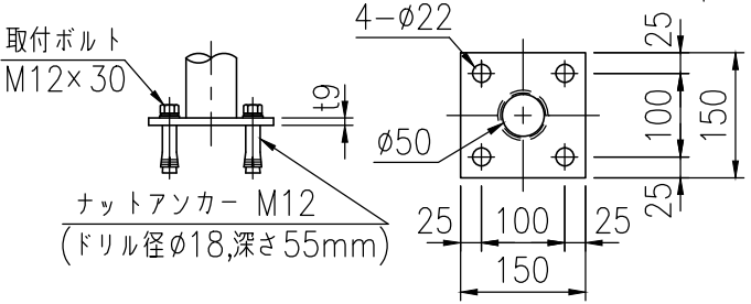
ベースプレート詳細図 (1/10)
