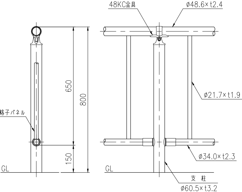
支柱図 (1/10)
