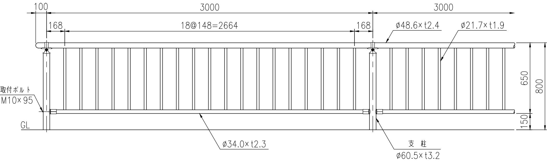
設置図 (1/20)
