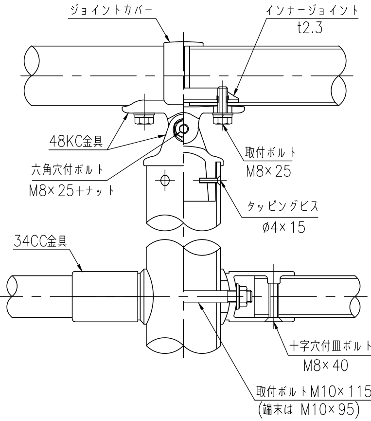
取付部詳細図 (1/3)
